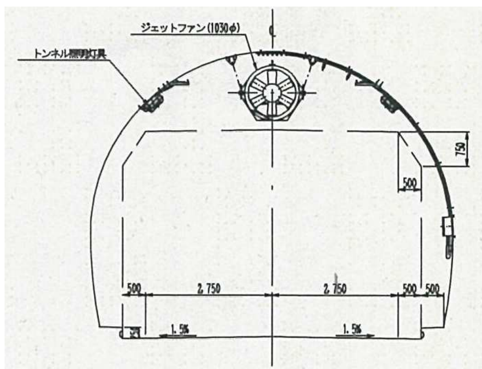
三才山トンネル断面図
