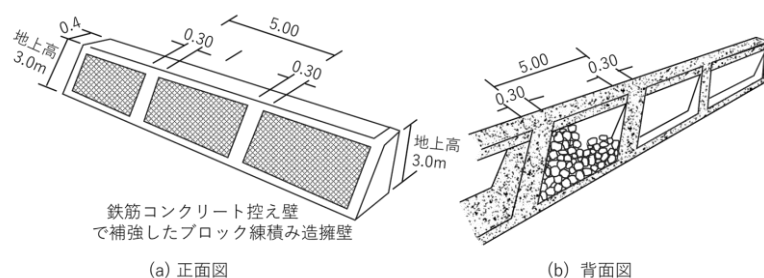
図 2.31 鉄筋コンクリート造控え壁の例
