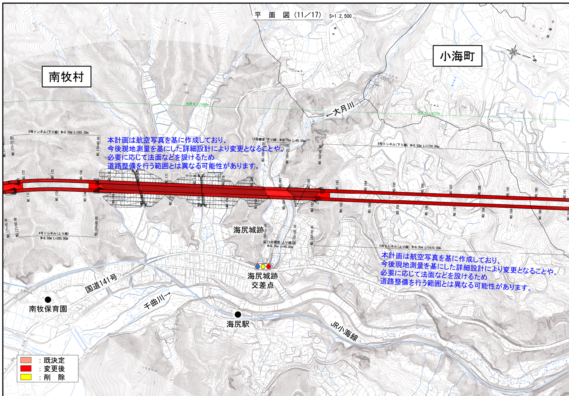
【計画平面図 (11/17)】
