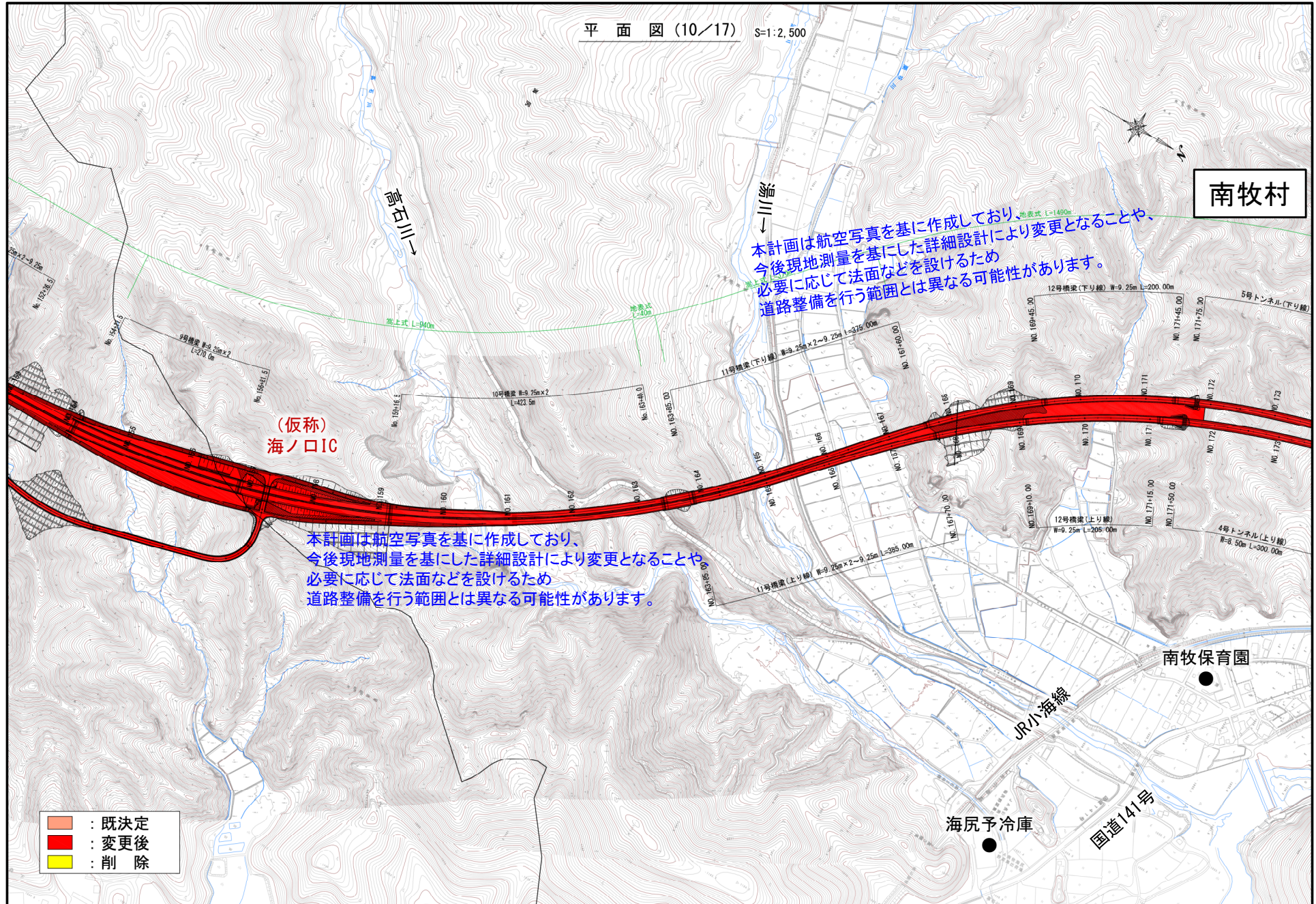
【計画平面図 (10/17)】
