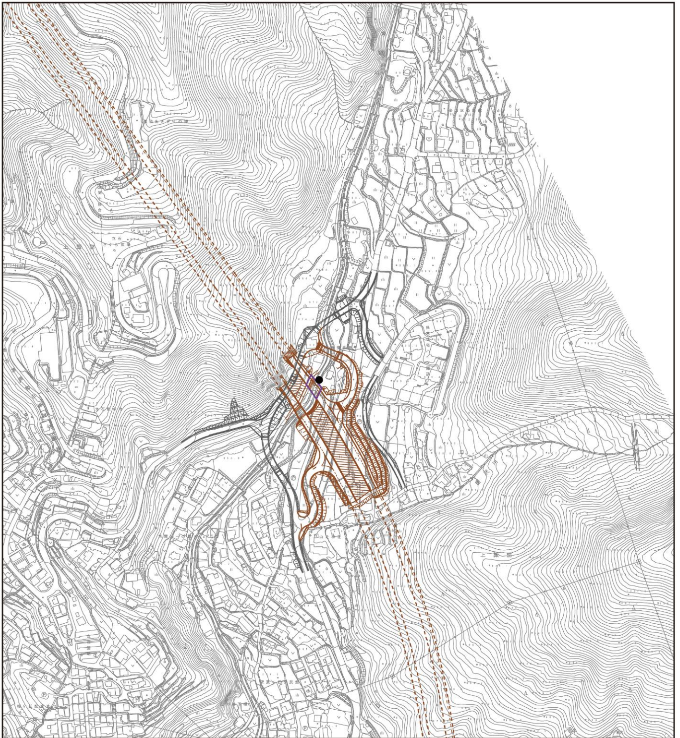
図 3.2.1 (8) 建設機械の稼働に係る騒音のユニット配置図 (8. 諏訪市上諏訪 4)
