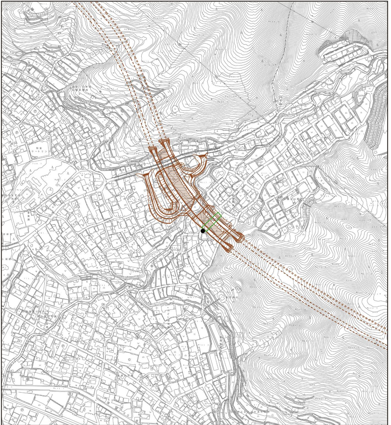
図 3.2.1 (12) 建設機械の稼働に係る騒音のユニット配置図 (12. 下諏訪町武居南 1)
