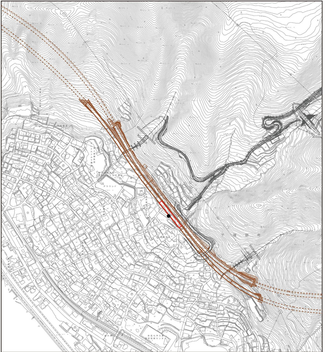
図 3.2.1 (10) 建設機械の稼働に係る騒音のユニット配置図 (10. 下諏訪町東高木 2)
