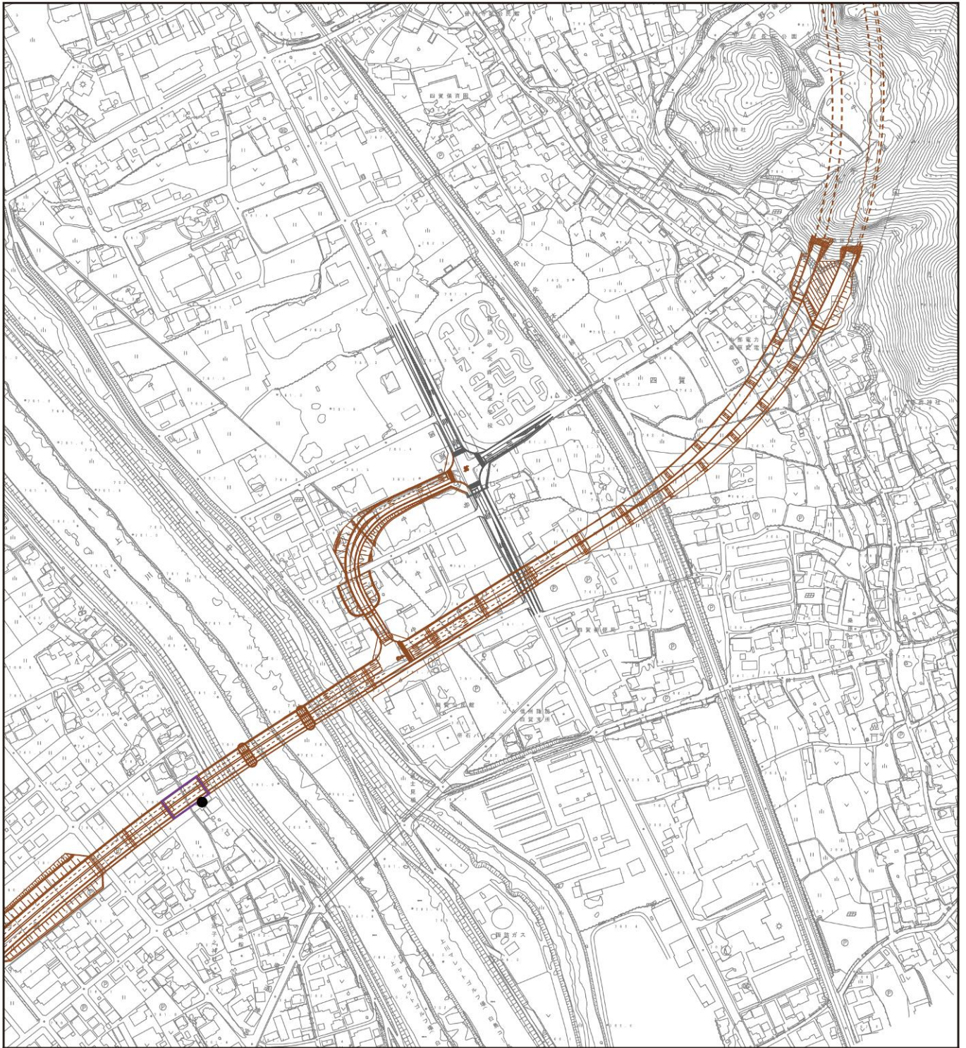
図 3.2.1 (3) 建設機械の稼働に係る騒音のユニット配置図 (3. 諏訪市四賀 3)
