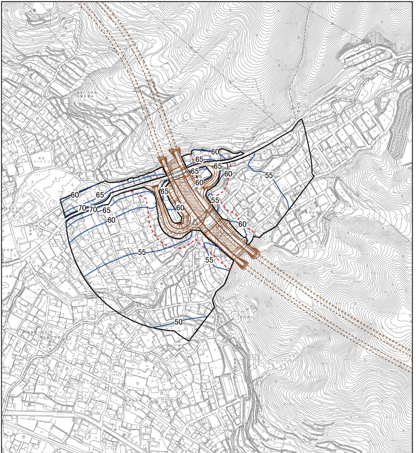
図 3.1.1 (21) 騒音分布図 (7. 下諏訪町武居南) 地上 1.2m 昼間
