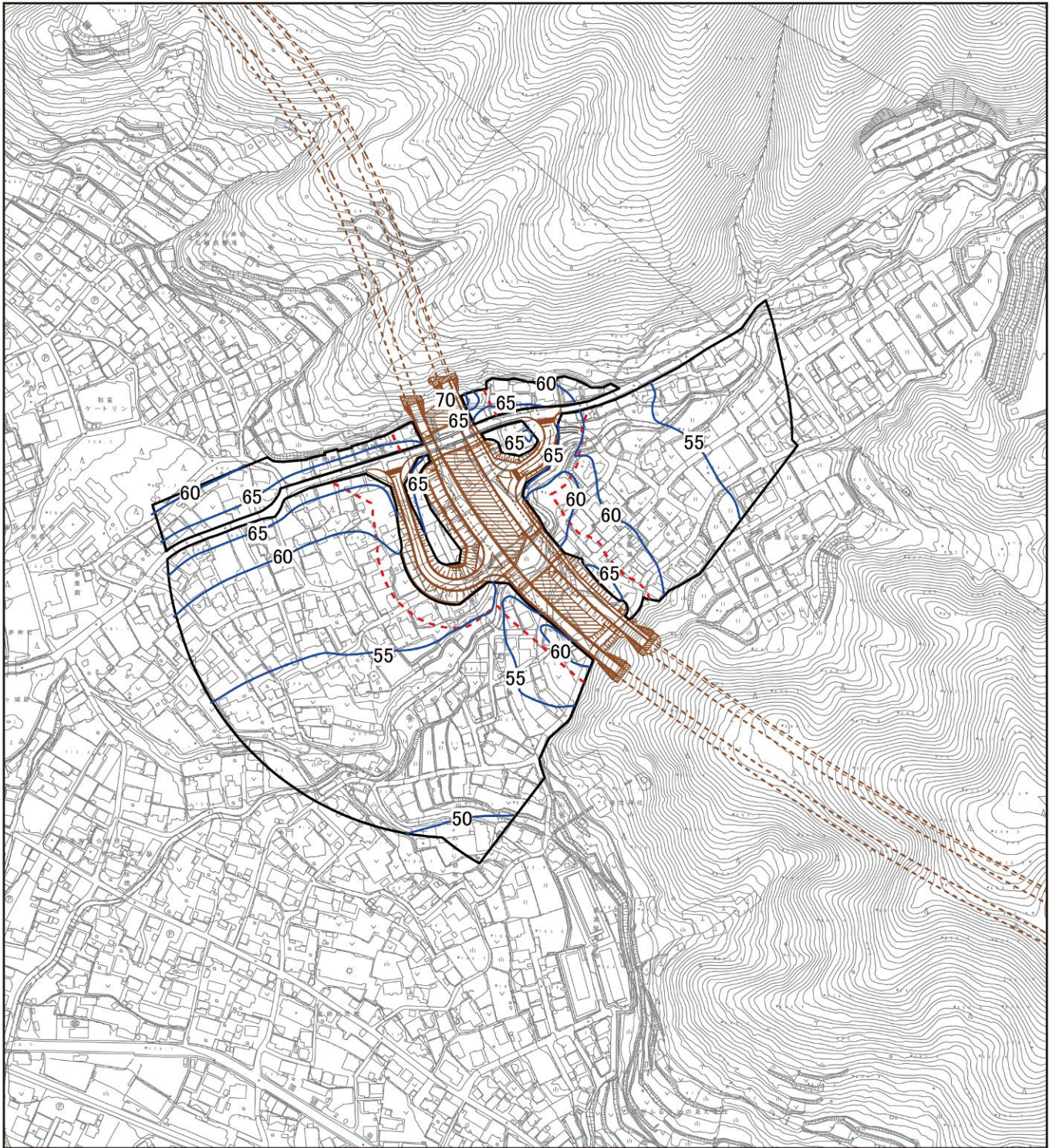
図 3.1.1 (22) 騒音分布図 (7. 下諏訪町武居南) 地上 4.2m 昼間
