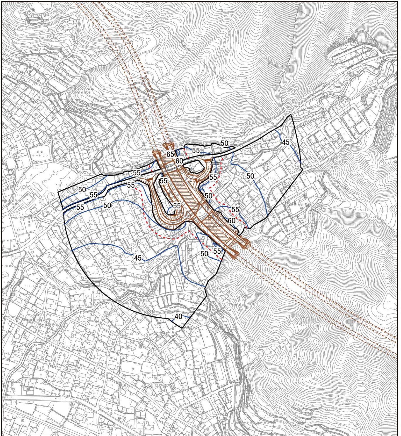
図 3.1.1 (24) 騒音分布図 (7.下諏訪町武居南) 地上 4.2m 夜間
