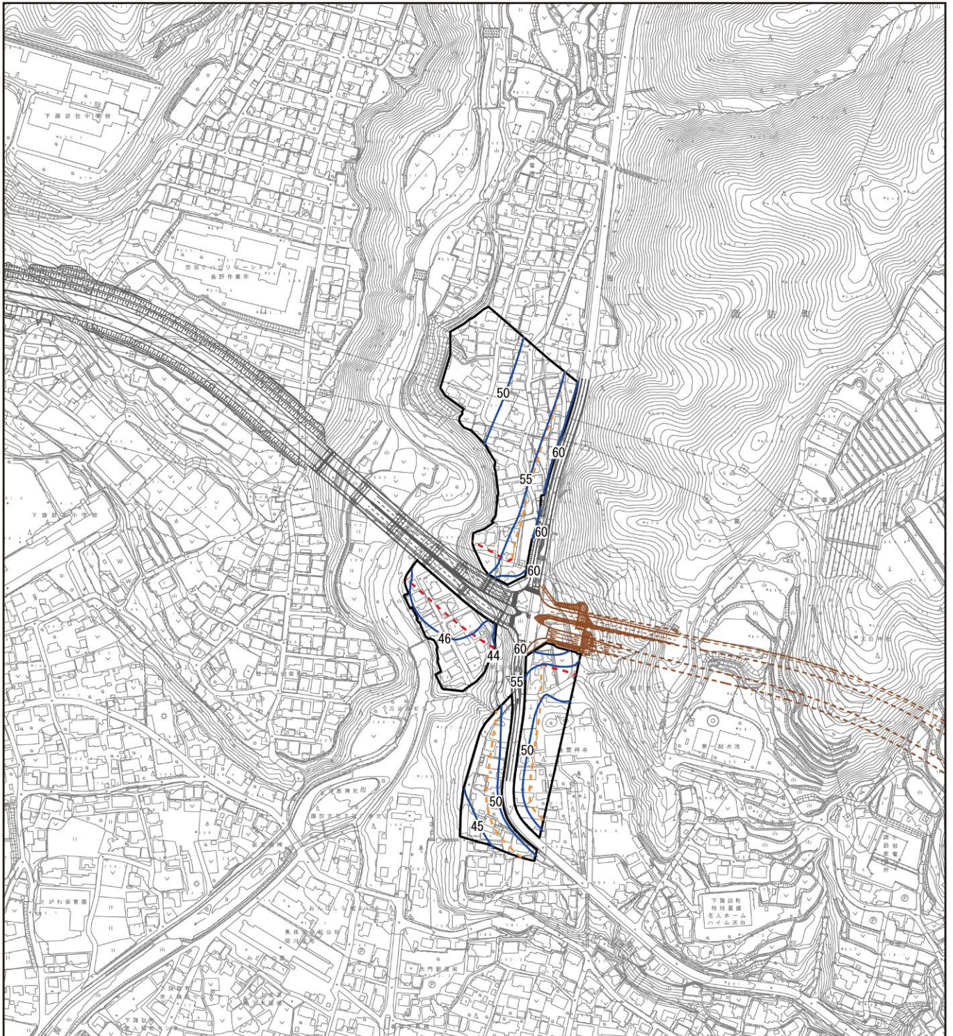
図 3.1.1 (27) 騒音分布図 (8. 下諏訪町東町中) 地上 1.2m 夜間
