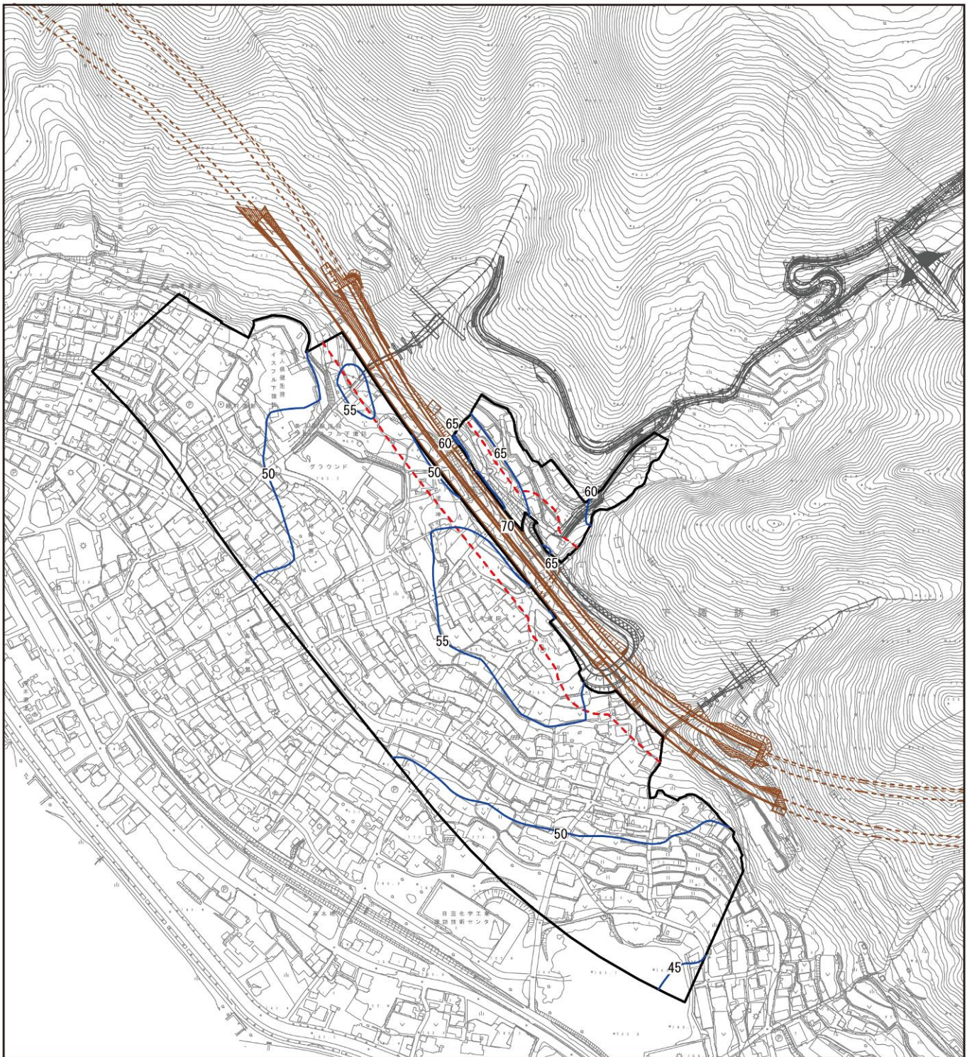
図 3.1.1 (17) 騒音分布図 (6. 下諏訪町東高木) 地上 1.2m 屋間
