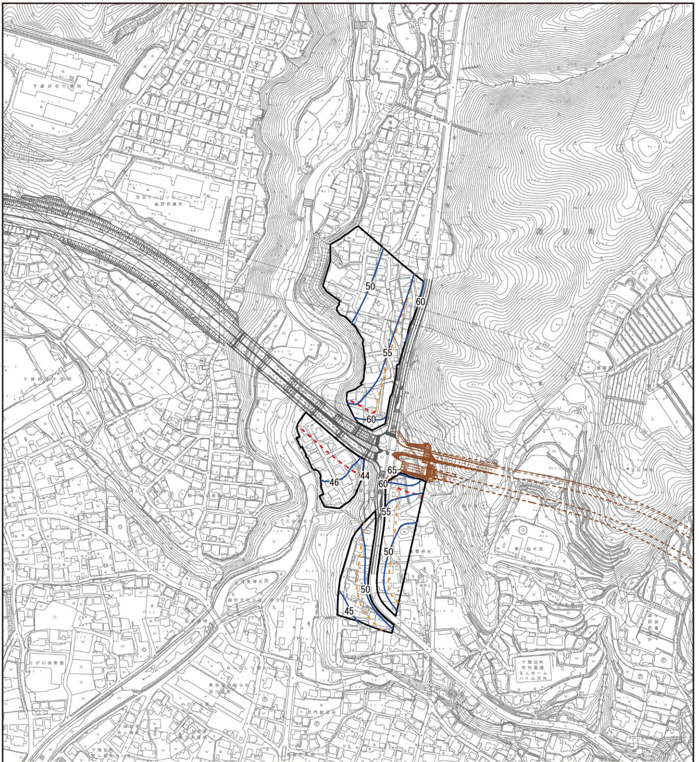
図 3.1.1 (28) 騒音分布図 (8. 下諏訪町東町中) 地上 4.2m 夜間
