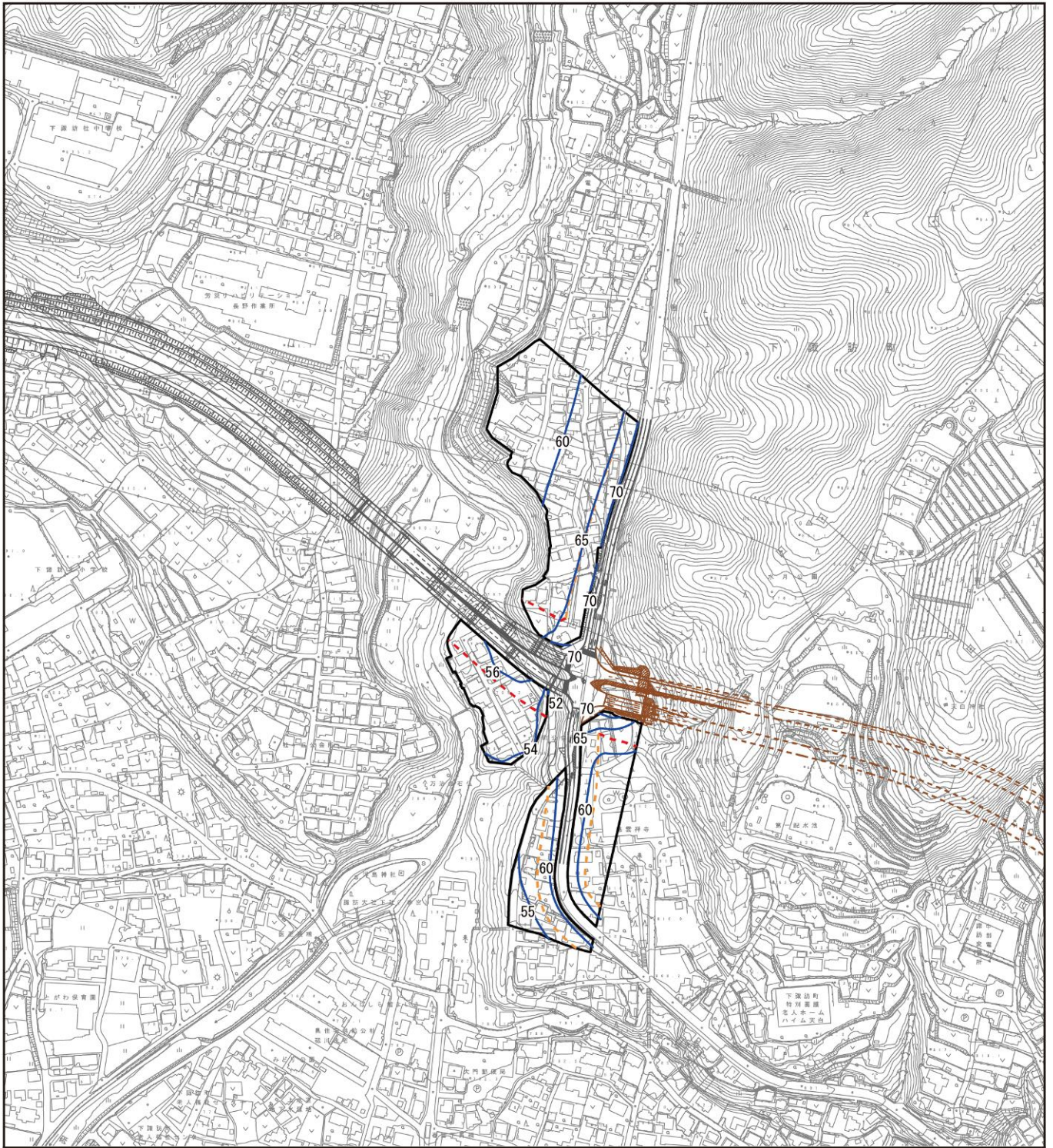
図 3.1.1 (25) 騒音分布図 (8.下諏訪町東町中) 地上 1.2m 屋間
