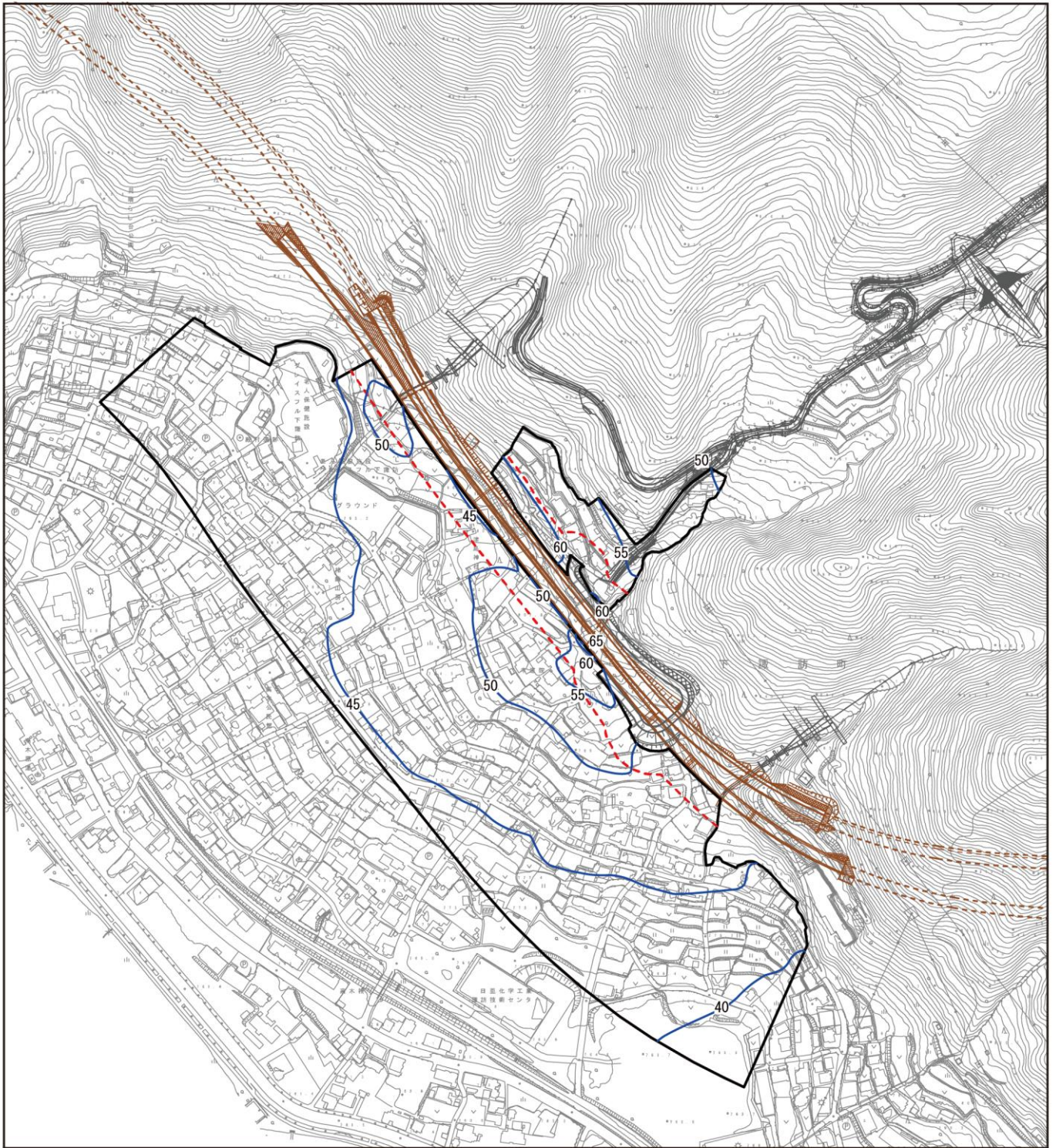
図 3.1.1 (19) 騒音分布図 (6. 下諏訪町東高木) 地上 1.2m 夜間
