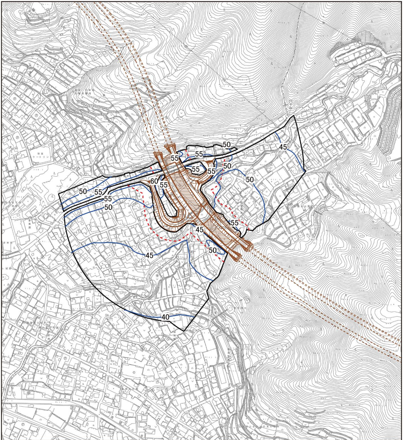
図 3.1.1 (23) 騒音分布図 (7. 下諏訪町武居南) 地上 1.2m 夜間
