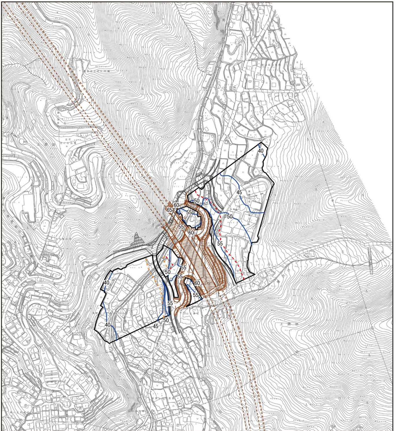
図 3.1.1 (15) 騒音分布図 (5. 諏訪市上諏訪) 地上 1.2m 夜間
