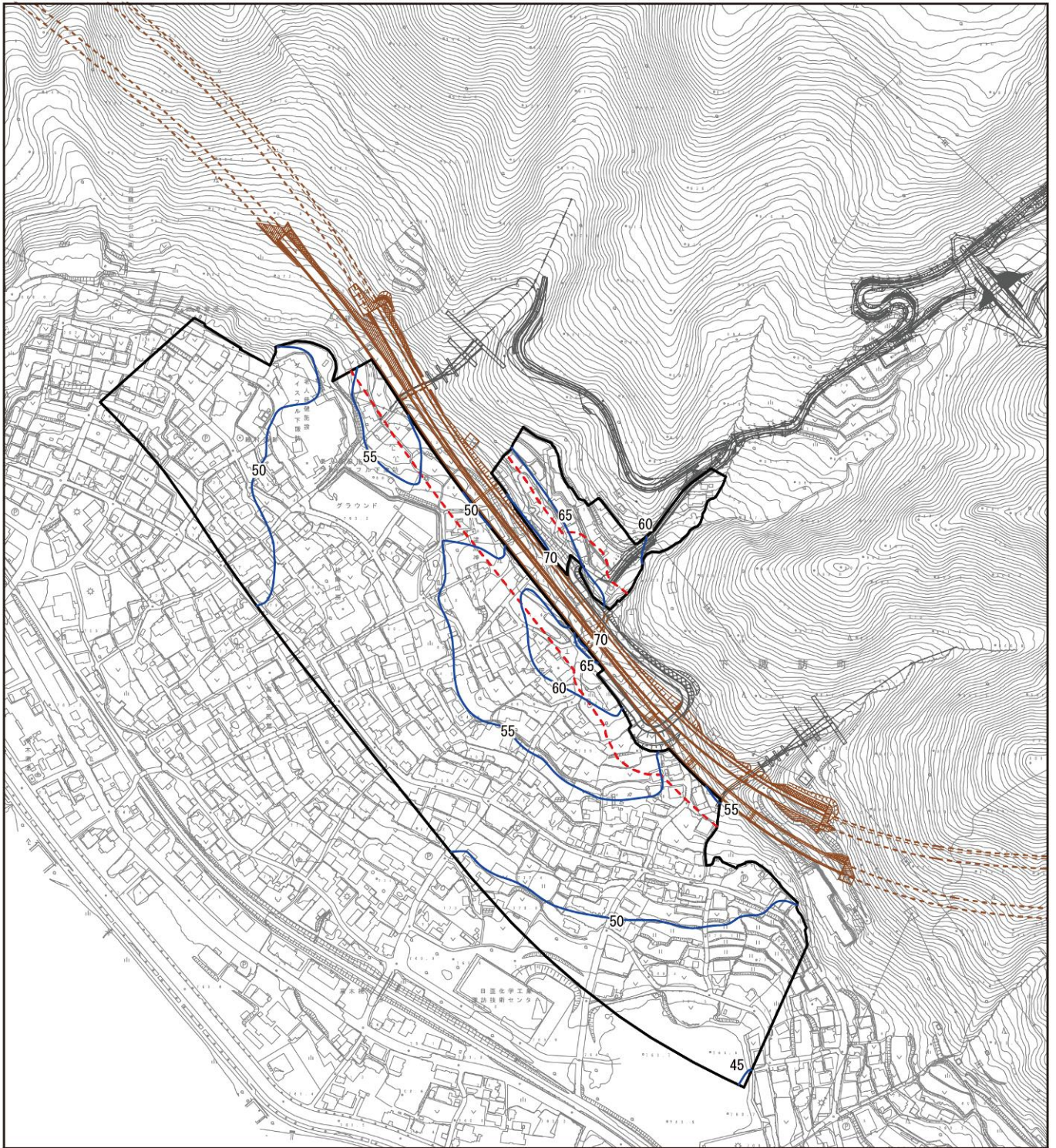
図 3.1.1 (18) 騒音分布図 (6. 下諏訪町東高木) 地上 4.2m 昼間
