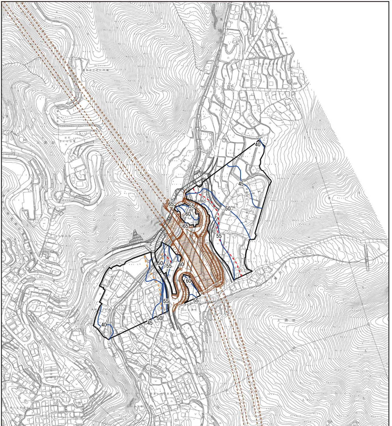
図 3.1.1 (16) 騒音分布図 (5. 諏訪市上諏訪) 地上 4.2m 夜間
