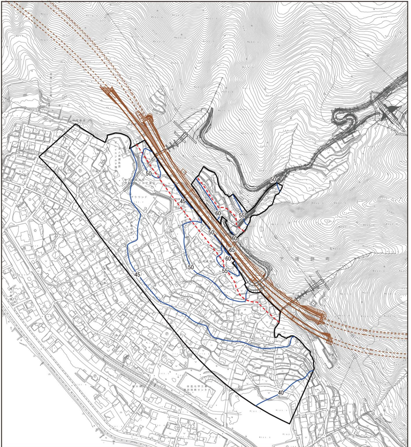
図 3.1.1 (20) 騒音分布図 (6. 下諏訪町東高木) 地上 4.2m 夜間
