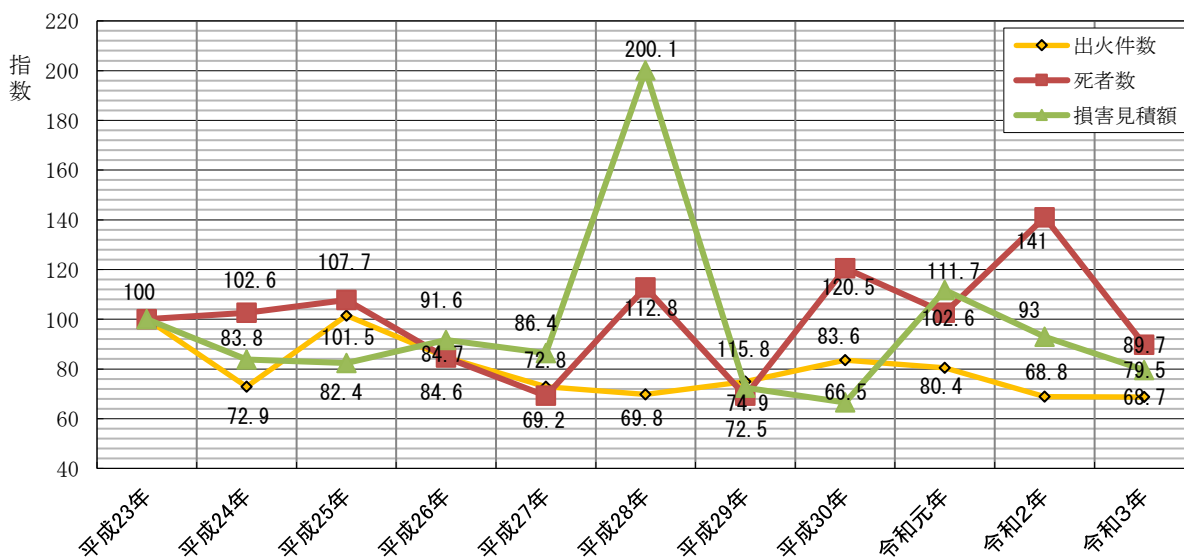
第 1 図 火 災 の 傾 向 (平成23年=100)
