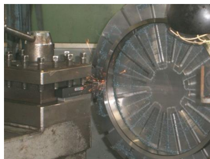
旋盤加工例
