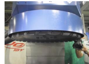
新開発したφ620mm切削工具(左)とφ150mm切削工具
