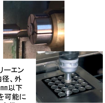
ロータリーエンコーダ スリット板加工技術
