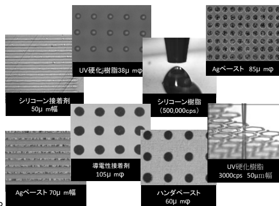
R-jet®による工業材料の塗布例
