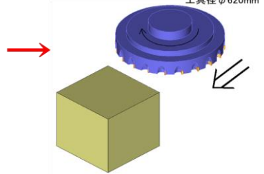
[新開発切削工具による新しい加工方法]
