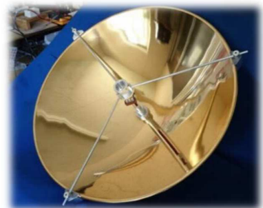
可视光通信实验局反射镜（镀金镜面）
