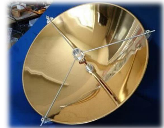
可視光通信実験局の反射鏡（鏡面金めっき）
