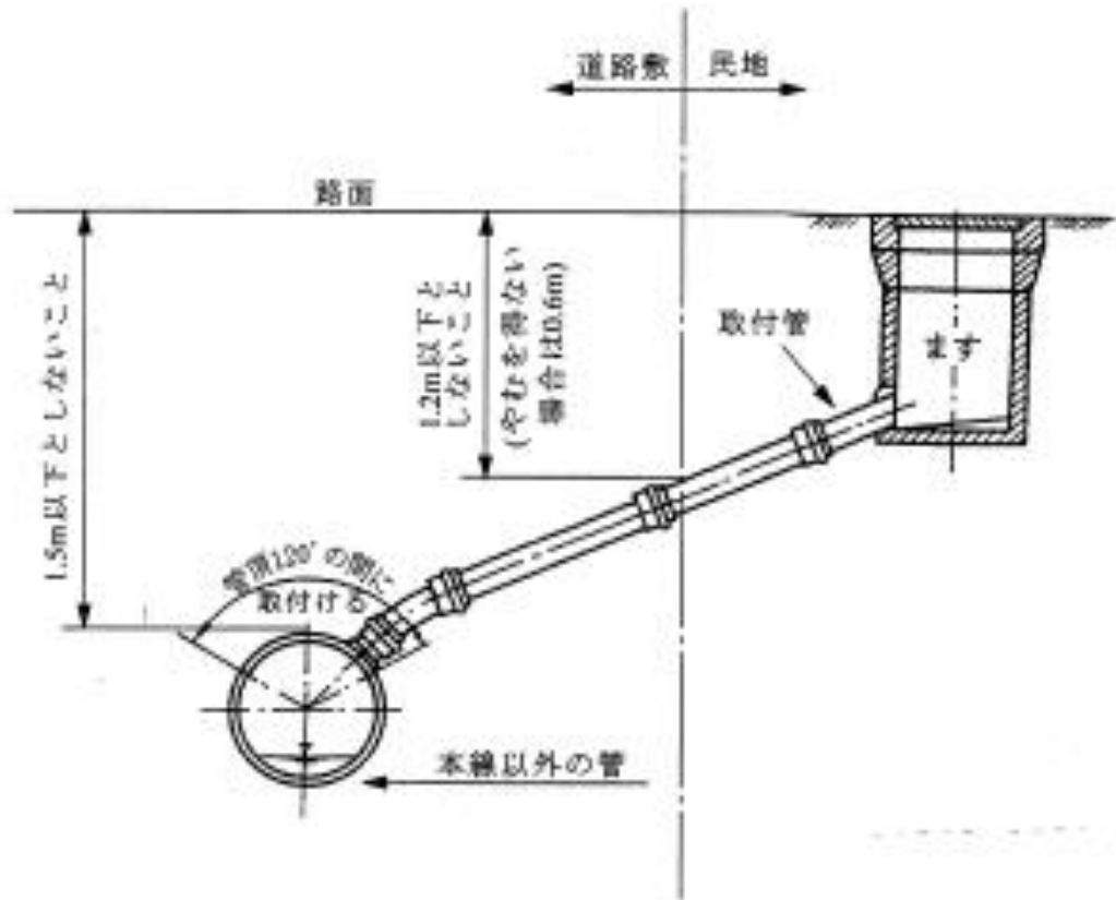
第 29(5)による下水道管の道路埋設例
