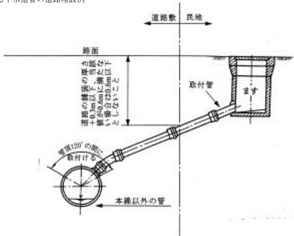
第 29(7)による下水道管の道路埋設例
