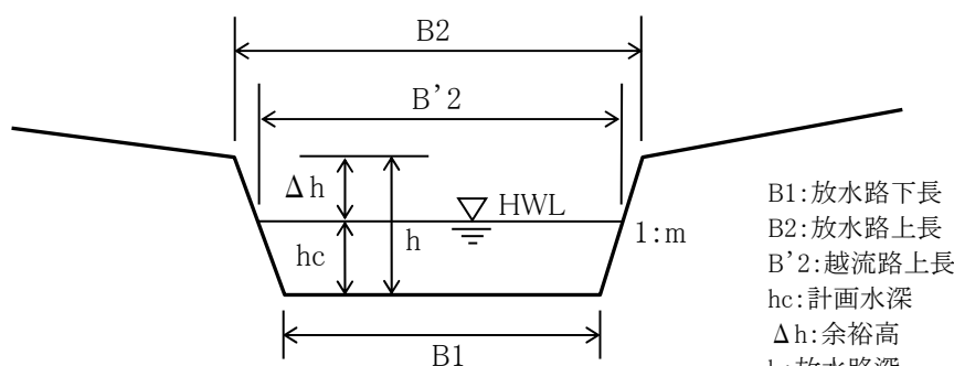
図 2-6 放水路断面の諸元
