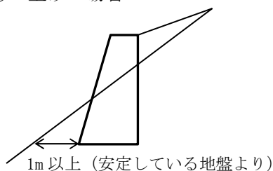
図 6－9 根入れ量
