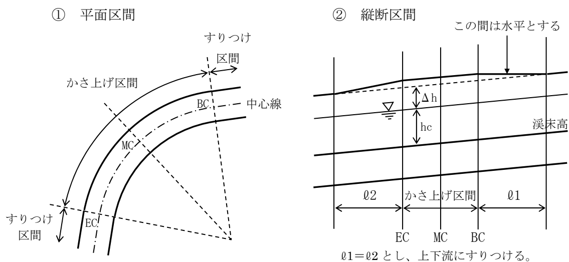
図 5-5 かさ上げ区間
