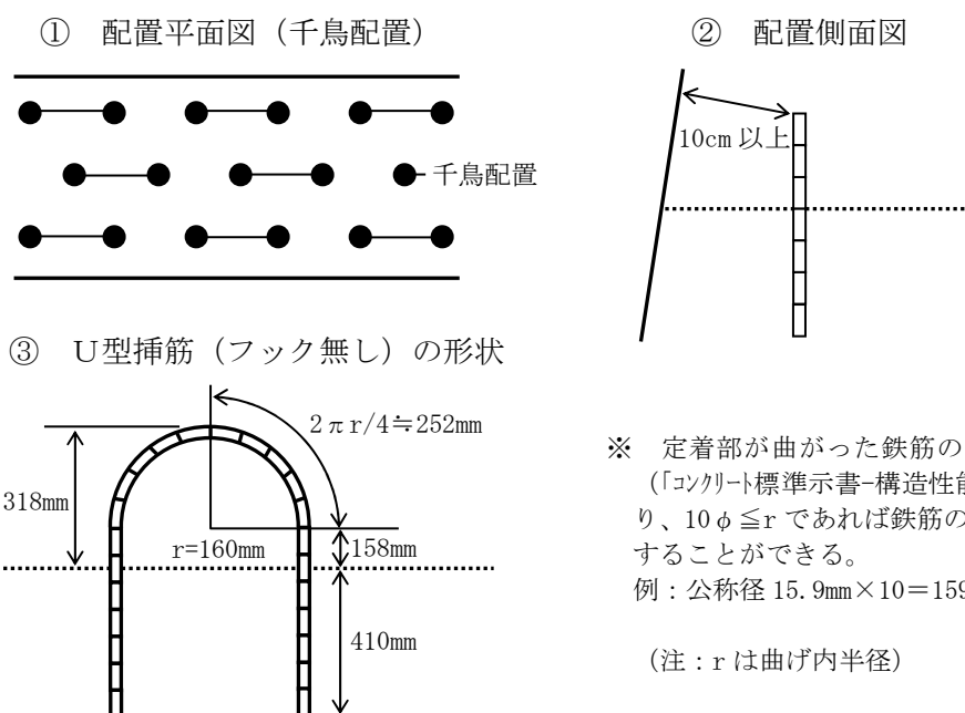
図 2-2-4 挿し筋の標準構造
