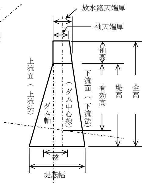
図 2-3 側面図
