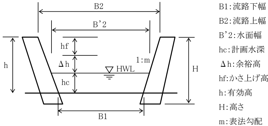
図 5-4 流路断面の諸元
