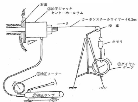
図4-3 引抜試験概要図
