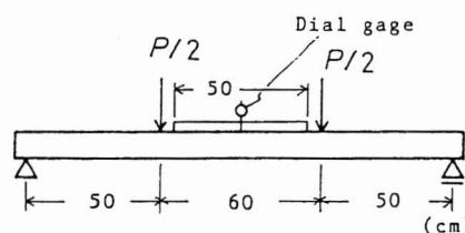
図-45 北海道試料での実大材曲げ試験 (小泉ら (52) 原図) Method of bending test in Hokkaido. (KOIZUMI et al(52))
