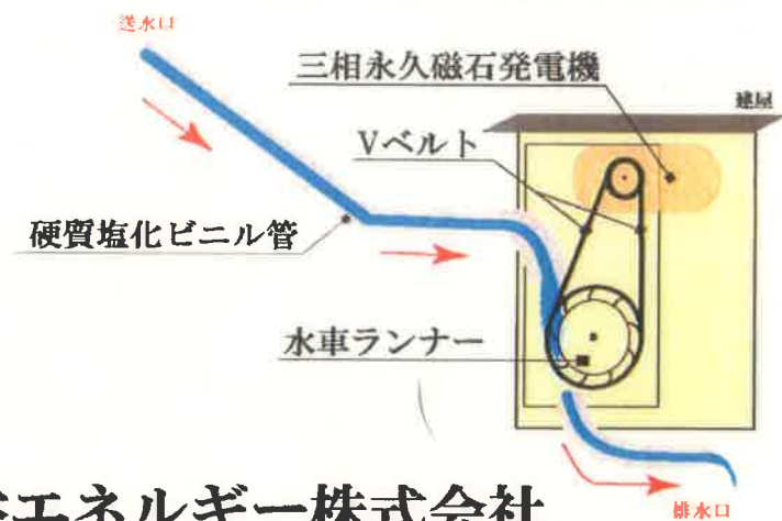
[小水力発電構造断面図]
