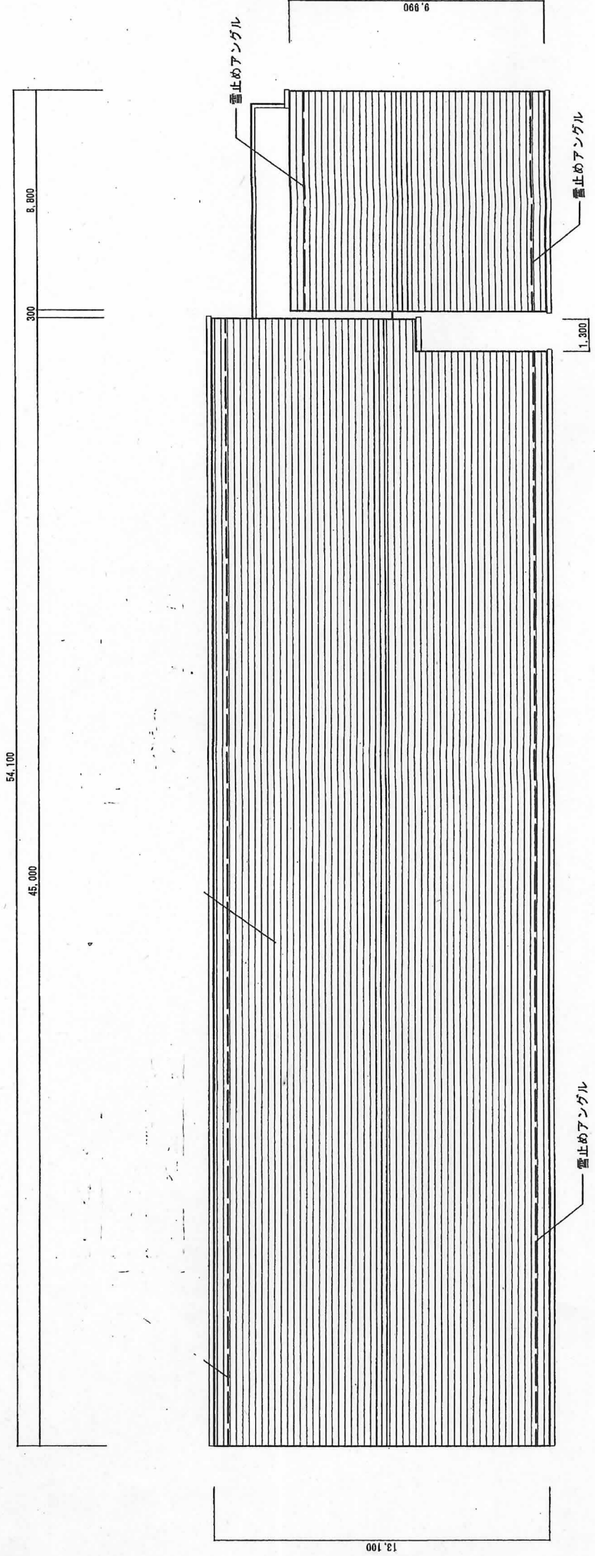
住宅棟 屋根伏図 1/200
