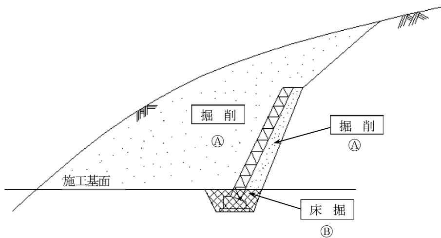
図2-17 逆T擁壁の場合
