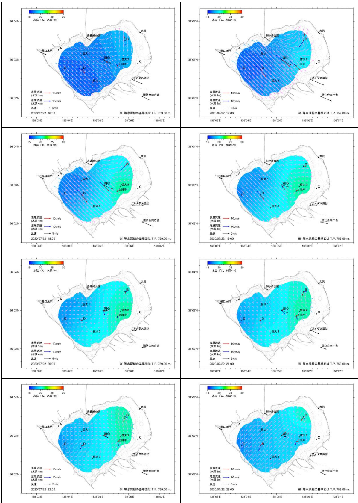
図 5.2(9) 湖内流況推定結果(2020年7月22日 16時~23時)
