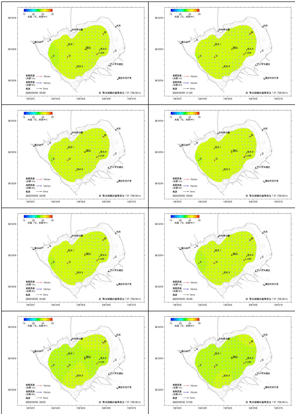
図 5.2(49) 湖内流況推定結果(2020年9月9日0時~7時)
