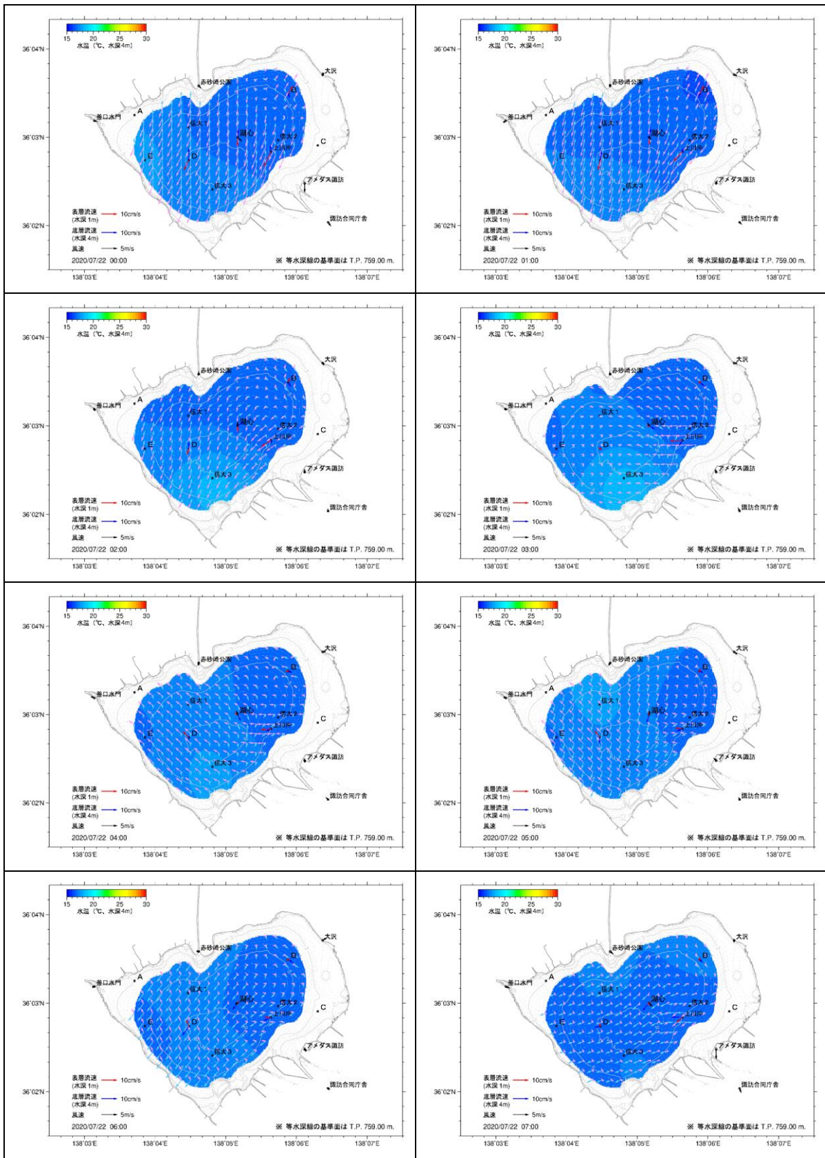
図 5.2(7) 湖内流況推定結果(2020年7月22日0時~7時)
