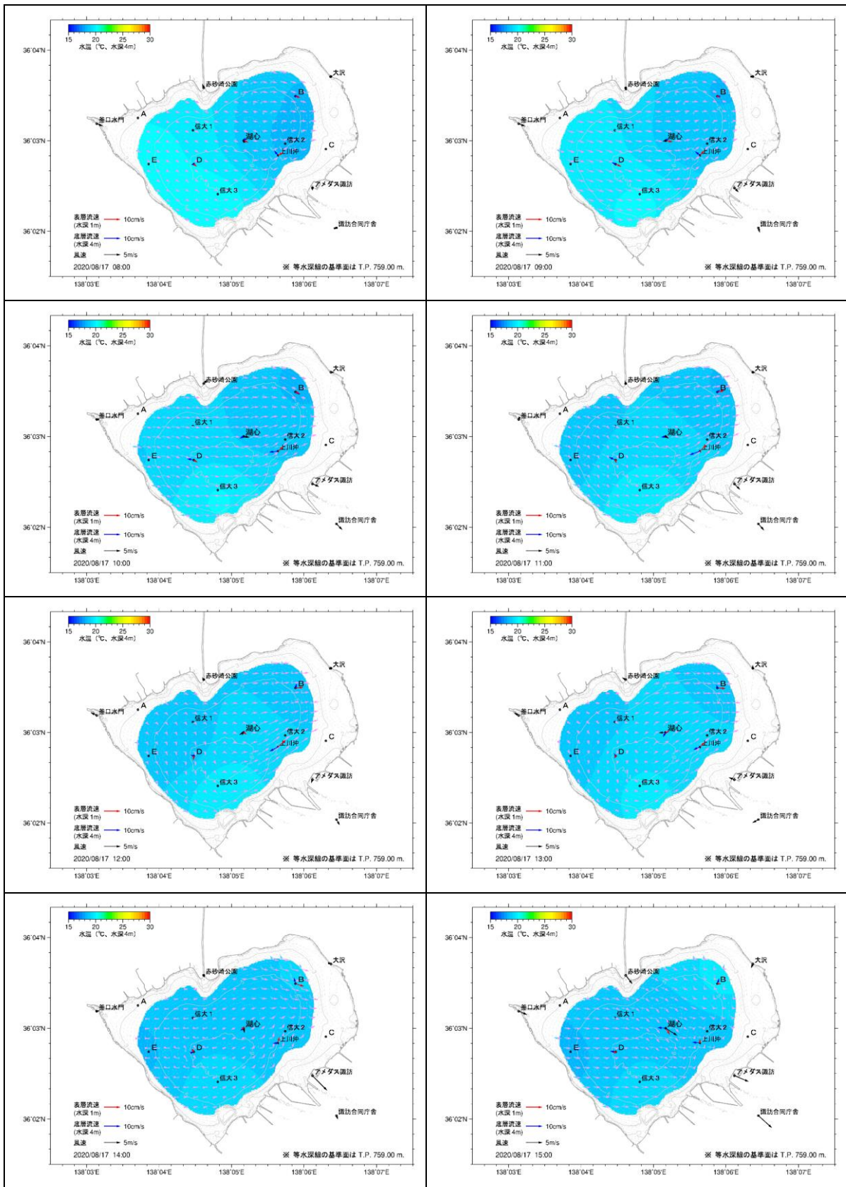
図 5.2(17) 湖内流況推定結果(2020年8月17日8時~15時)
