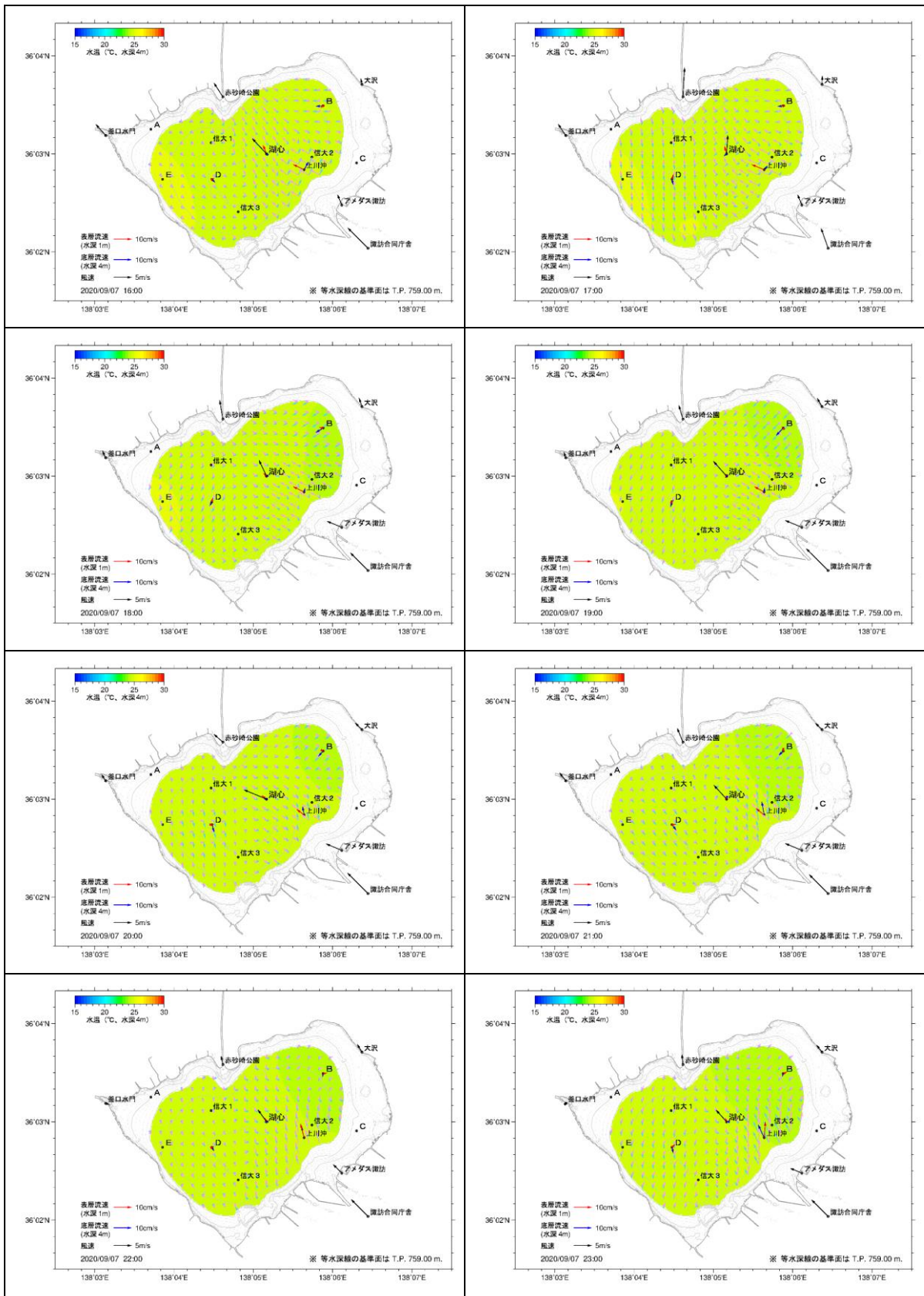
図 5.2(45) 湖内流況推定結果(2020年9月7日 16時~23時)
