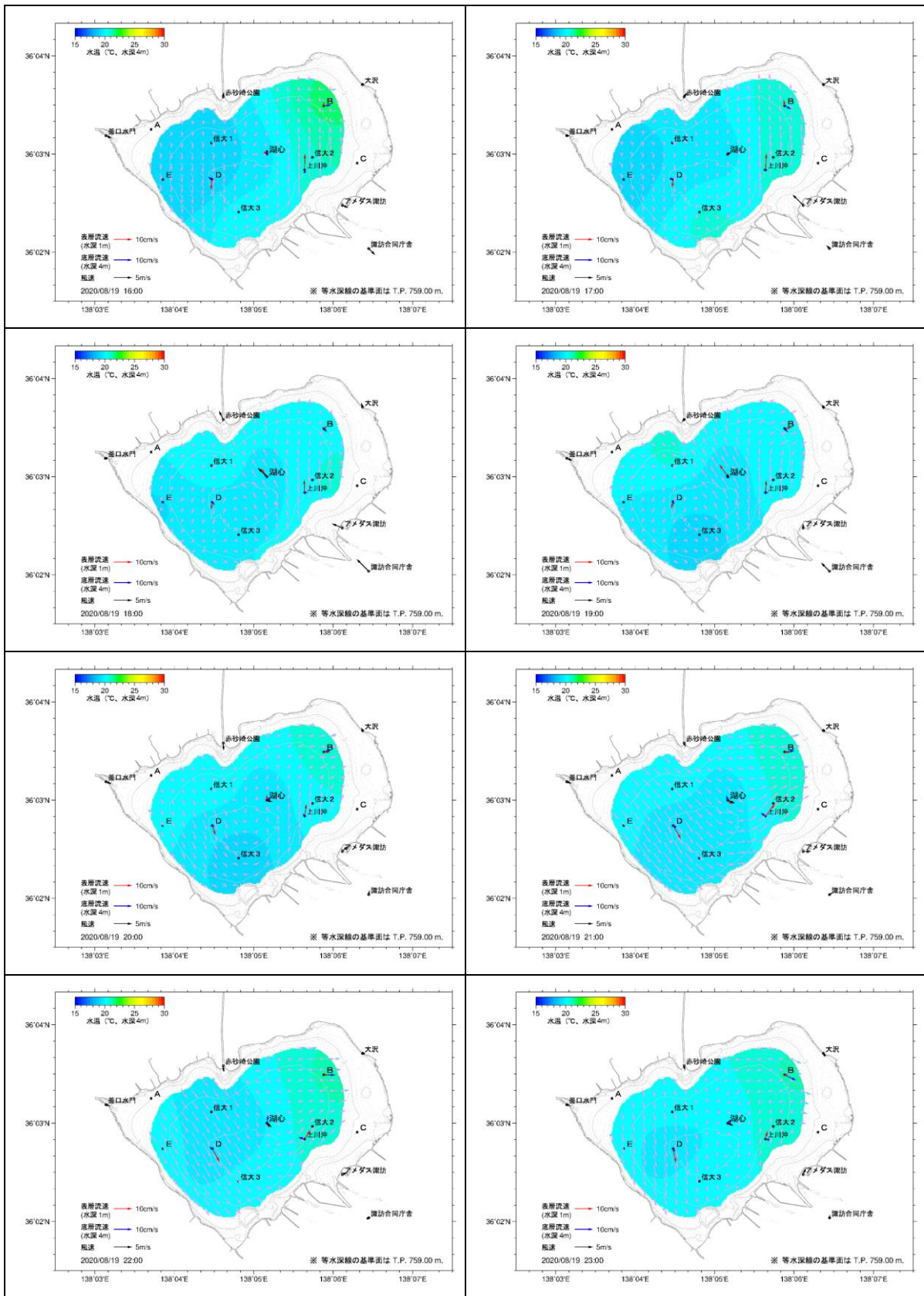
図 5.2(24) 湖内流況推定結果(2020年8月19日 16時~23時)
