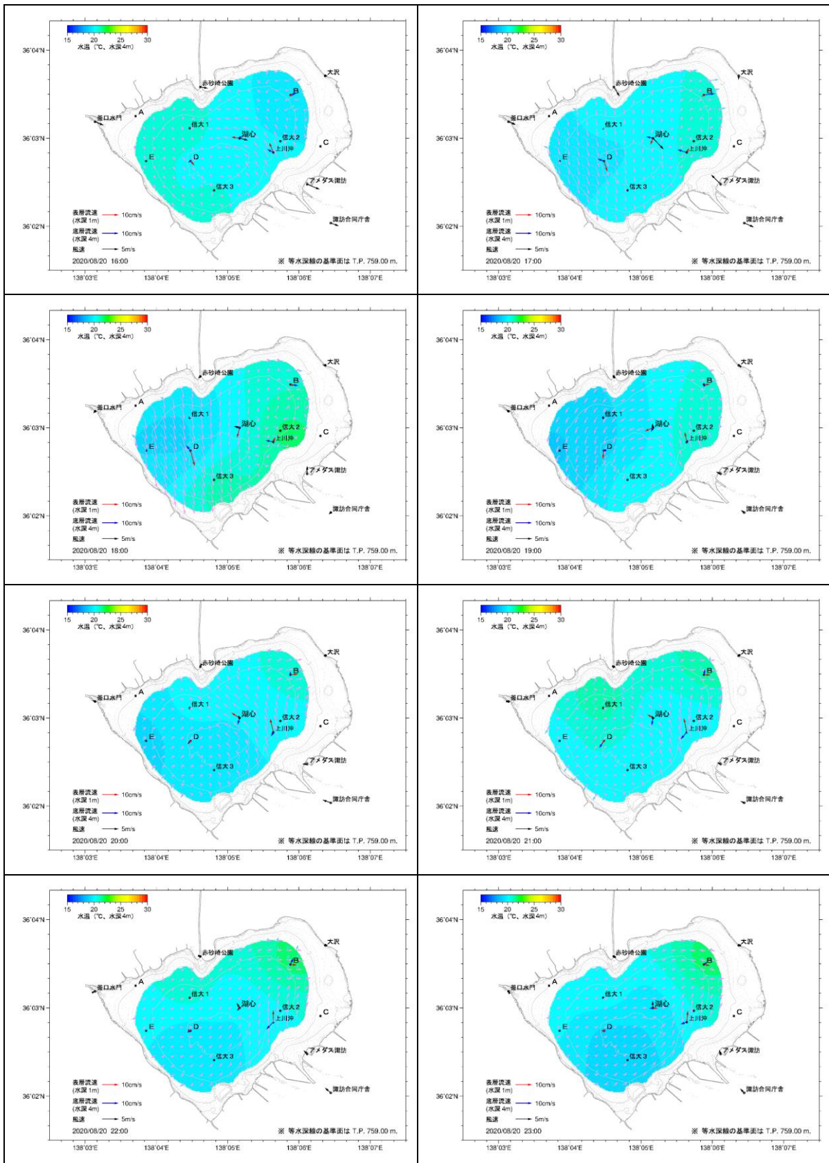
図 5.2(27) 湖内流況推定結果(2020年8月20日 16時~23時)
