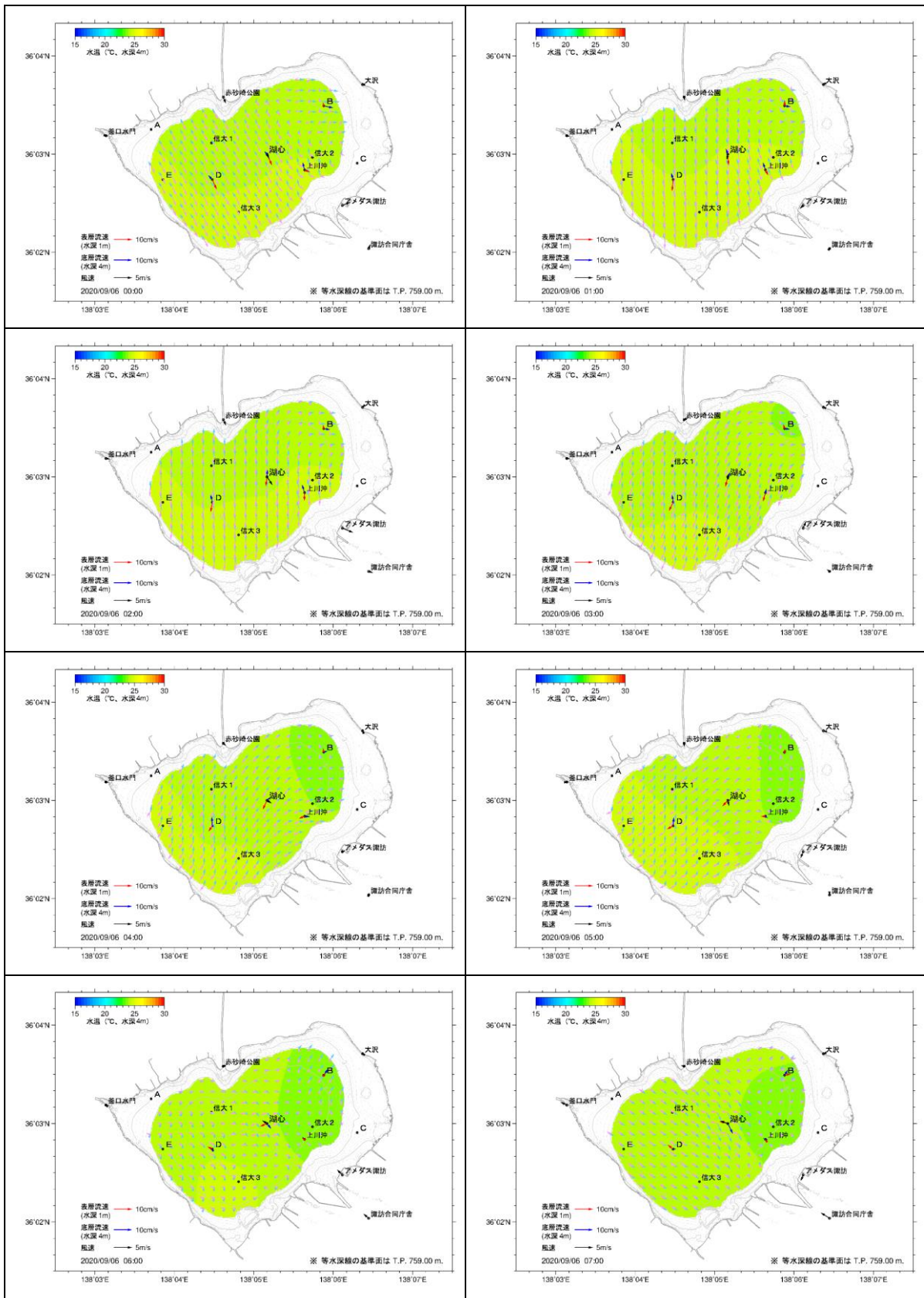
図 5.2(40) 湖内流況推定結果(2020年9月6日0時~7時)
