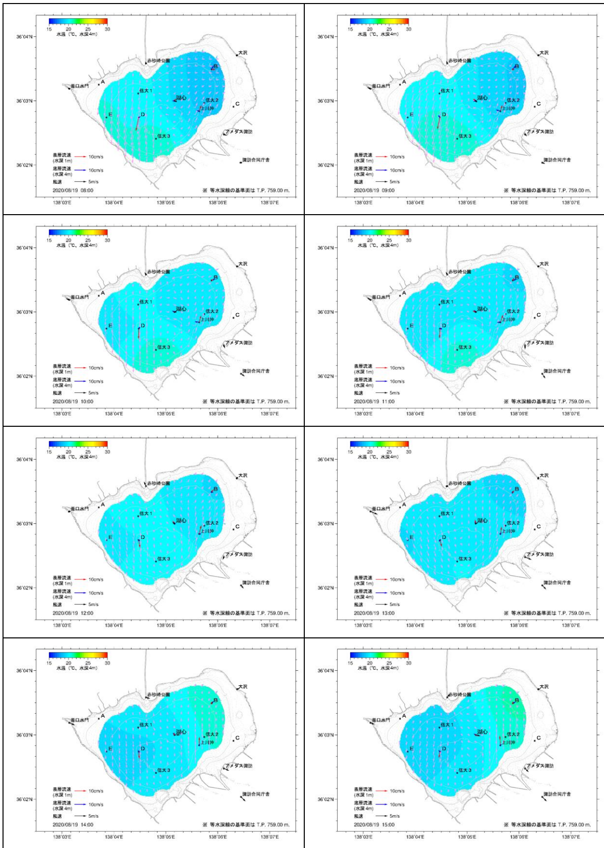
図 5.2(23) 湖内流況推定結果(2020年8月19日8時~15時)
