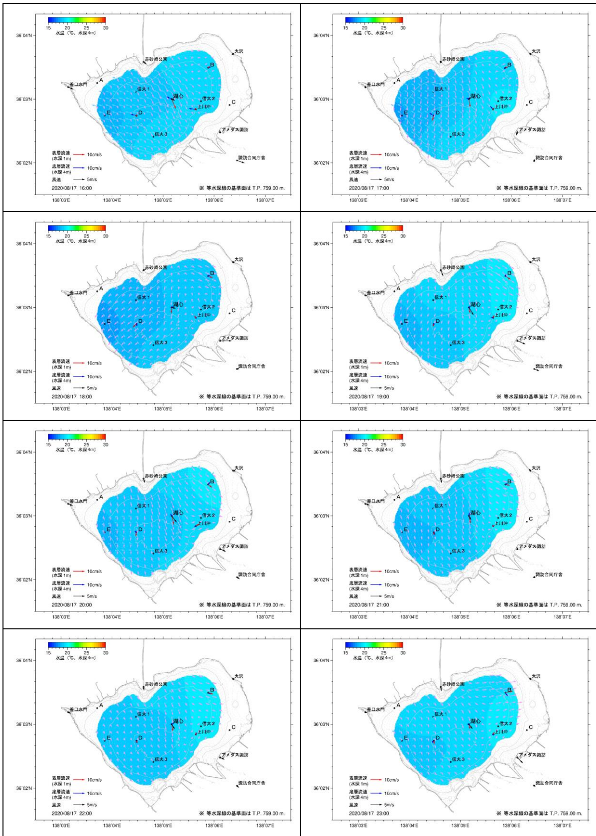
図 5.2(18) 湖内流況推定結果(2020年8月17日 16時~23時)
