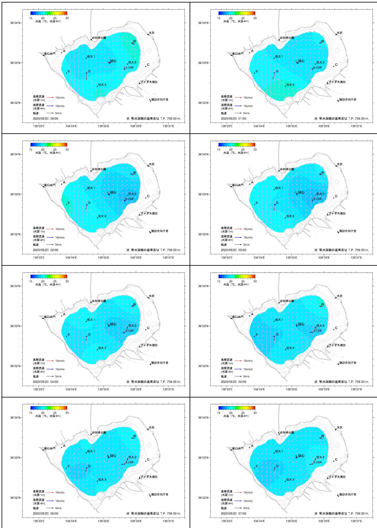
図 5.2(25) 湖内流況推定結果(2020年8月20日0時~7時)
