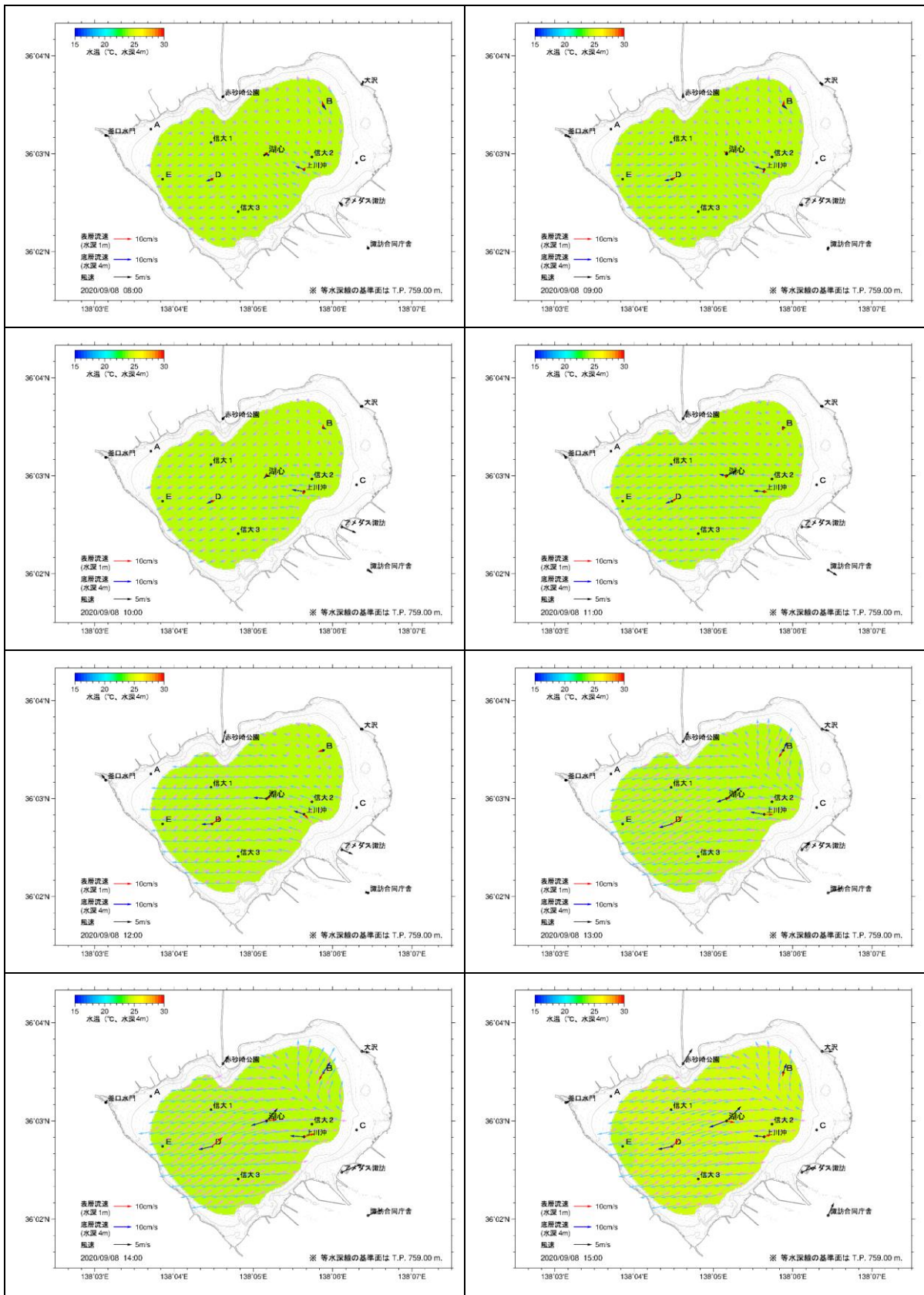
図 5.2(47) 湖内流況推定結果(2020年9月8日 8時~15時)
