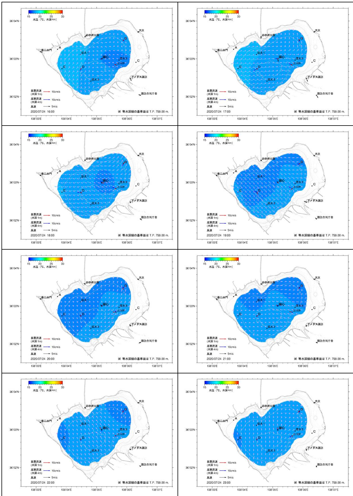
図 5.2(15) 湖内流況推定結果(2020年7月24日 16時~23時)
