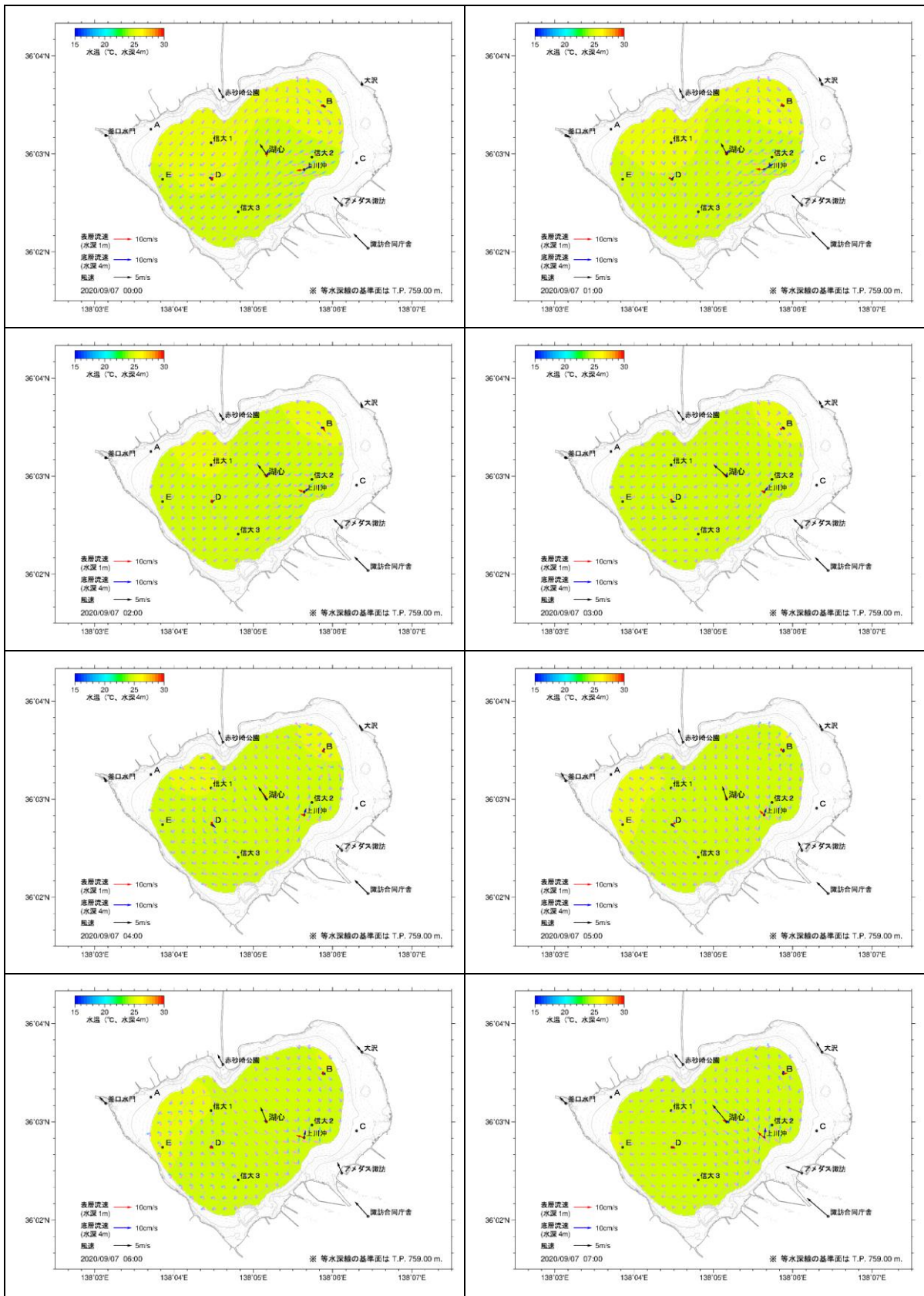
図 5.2(43) 湖内流況推定結果(2020年9月7日0時~7時)
