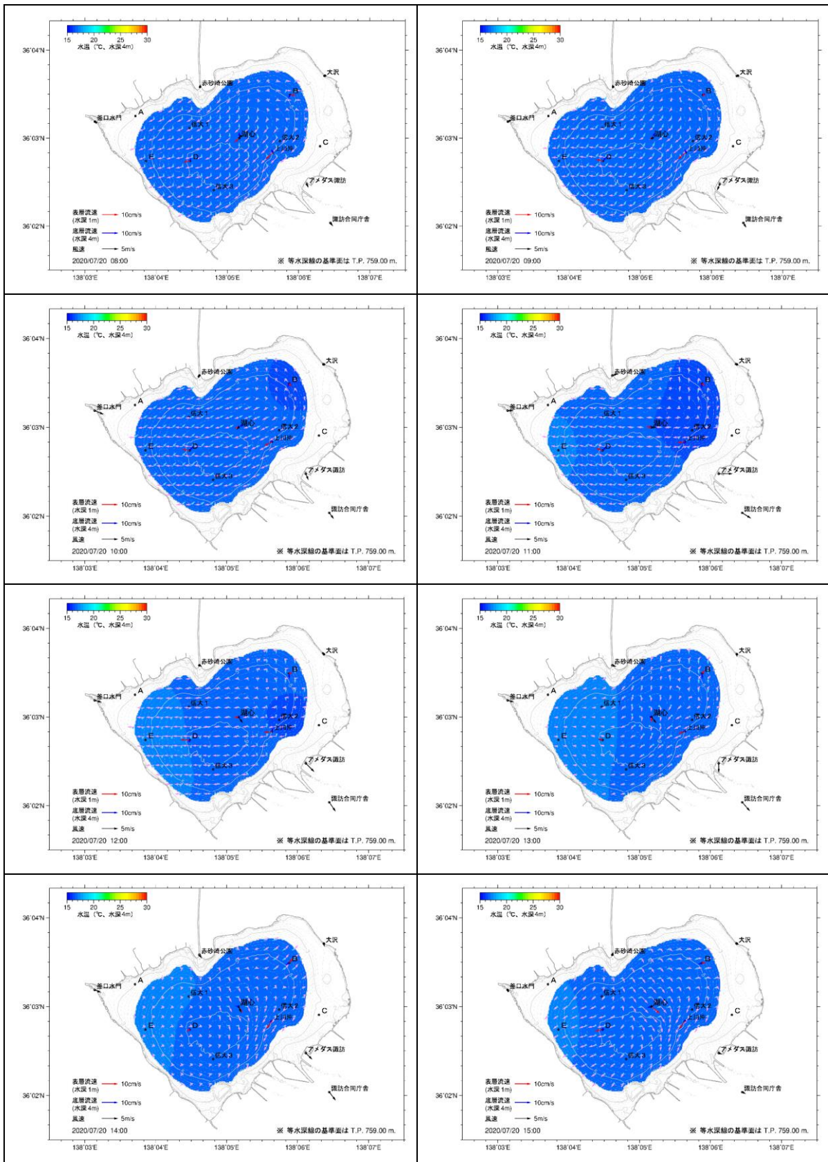
図 5.2(2) 湖内流況推定結果(2020年7月20日8時~15時)
