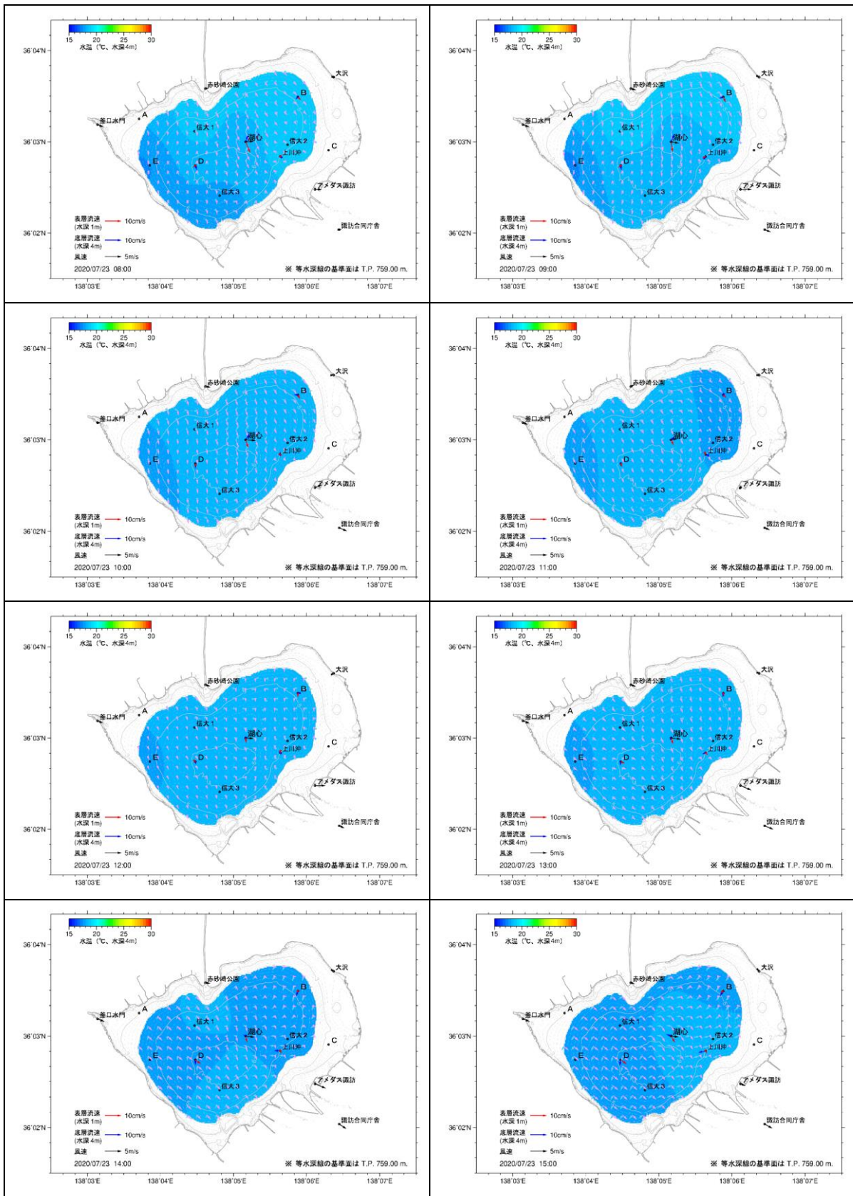
図 5.2(11) 湖内流況推定結果(2020年7月23日8時~15時)
