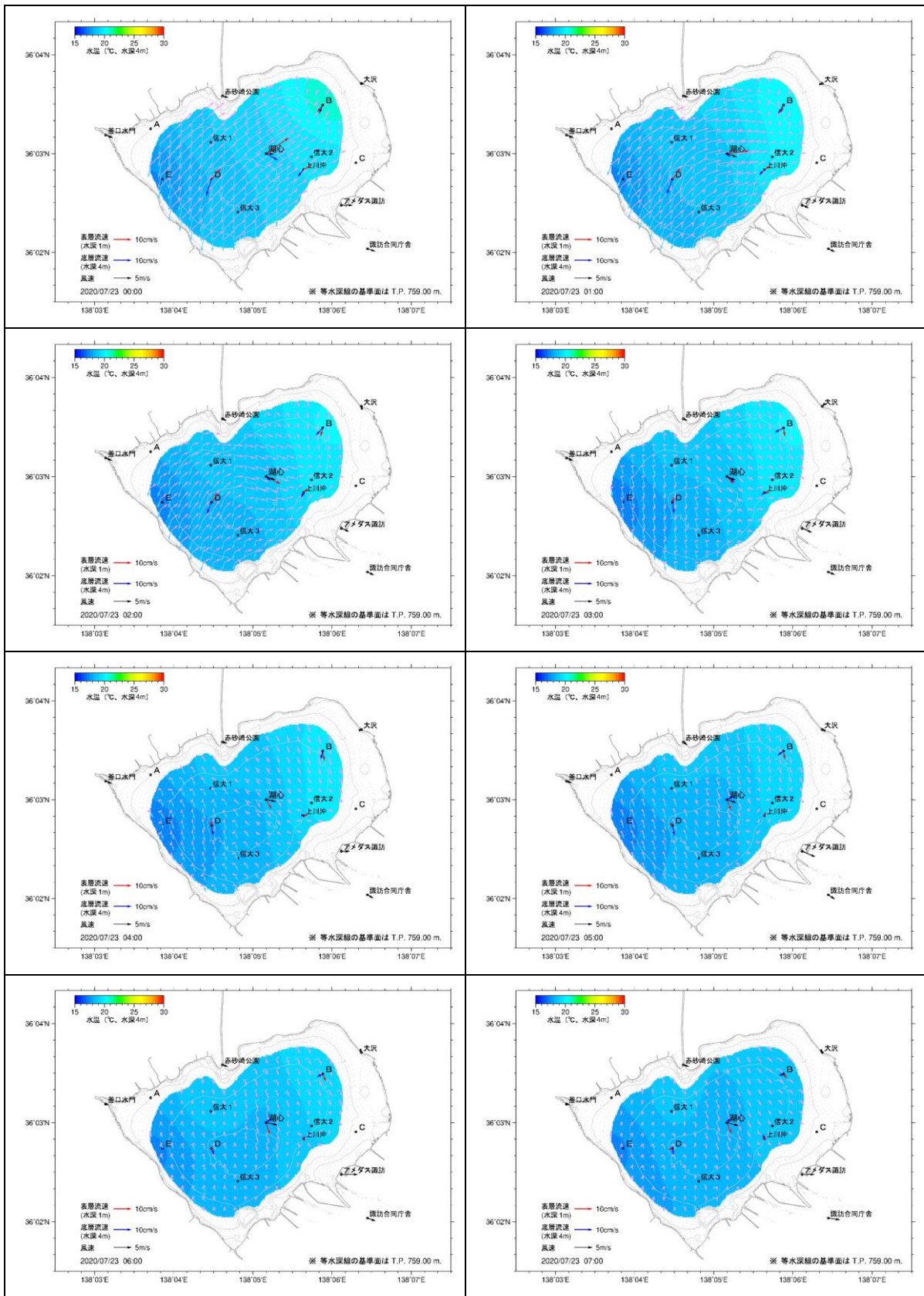
図 5.2(10) 湖内流況推定結果(2020年7月23日0時~7時)
