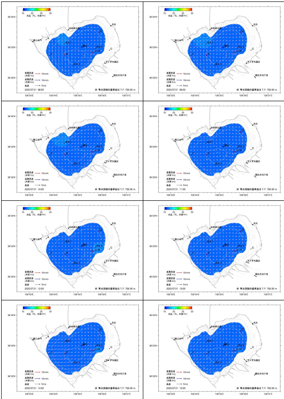
図 5.2(5) 湖内流況推定結果(2020年7月21日8時~15時)
