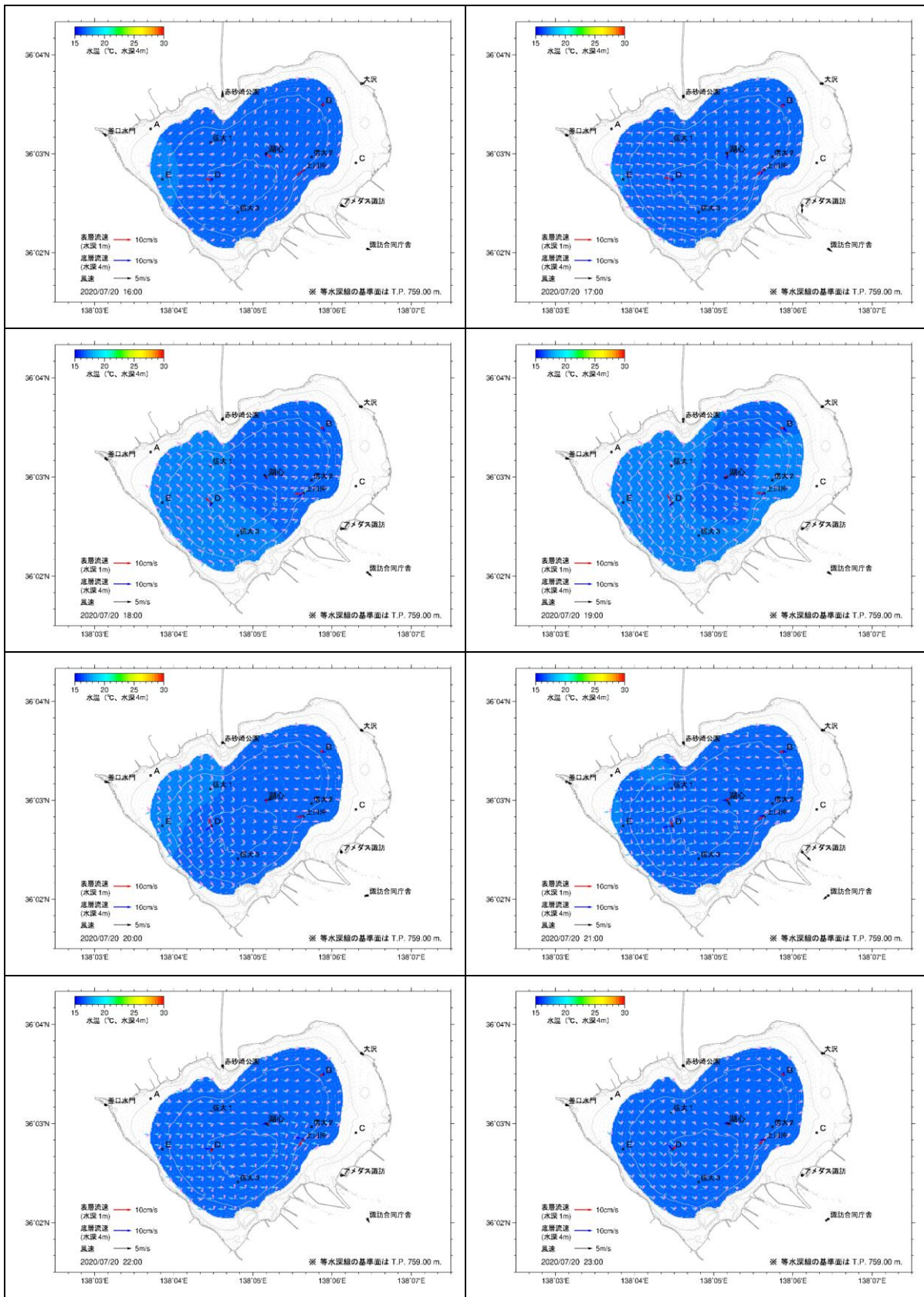
図 5.2(3) 湖内流況推定結果(2020年7月20日 16時~23時)
