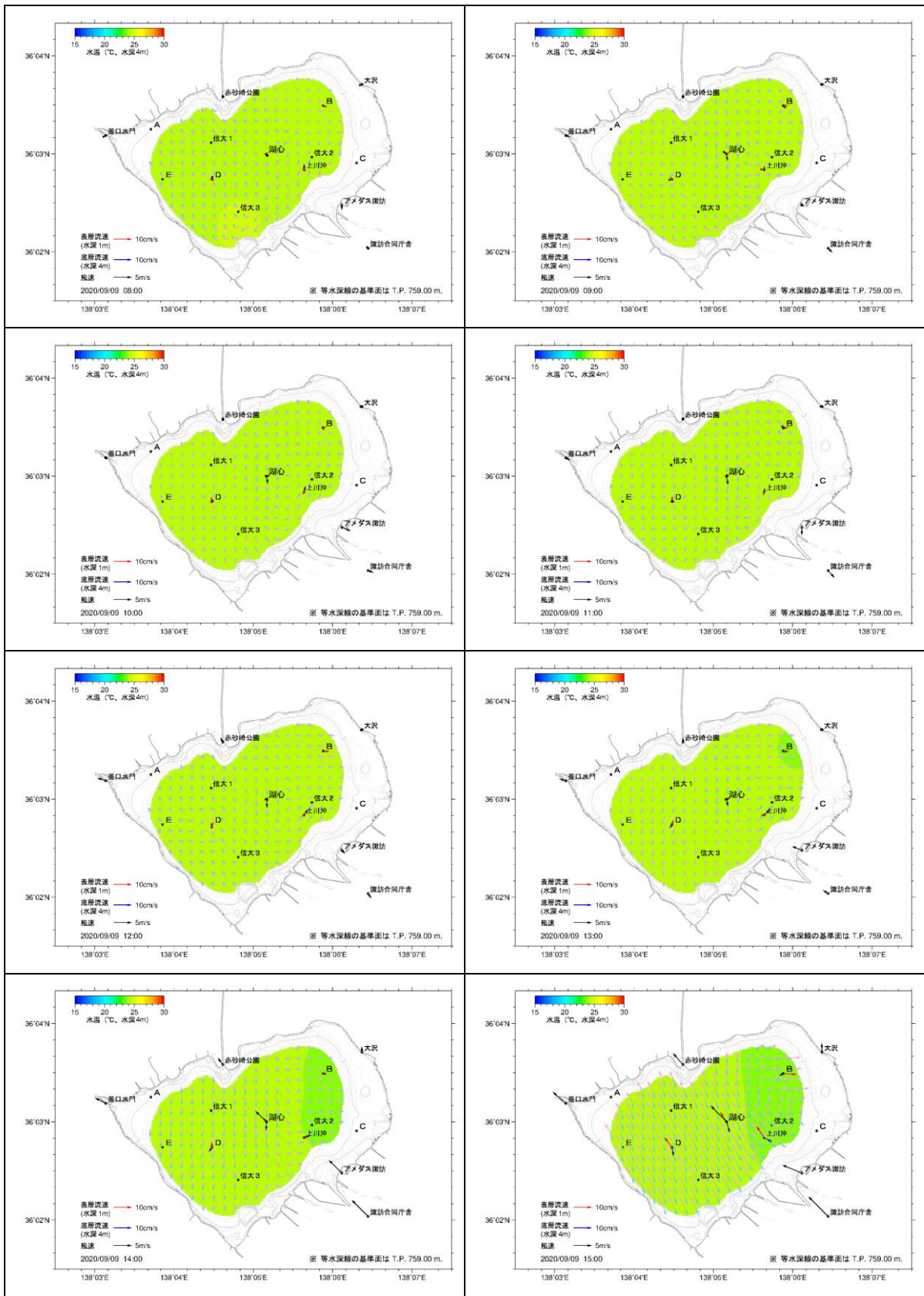
図 5.2(50) 湖内流況推定結果(2020年9月9日8時~15時)
