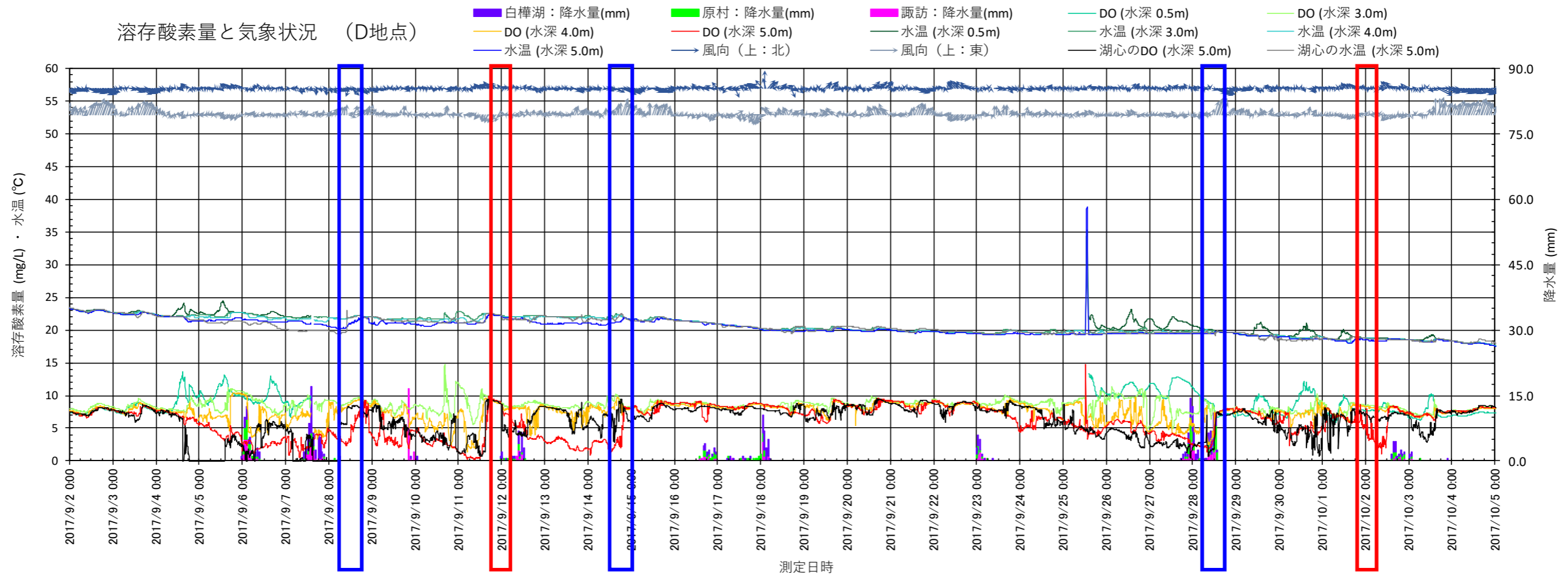
図 3.1.45 (2) 2017 (平成 29) 年度における溶存酸素量と気象状況 (D 地点)
