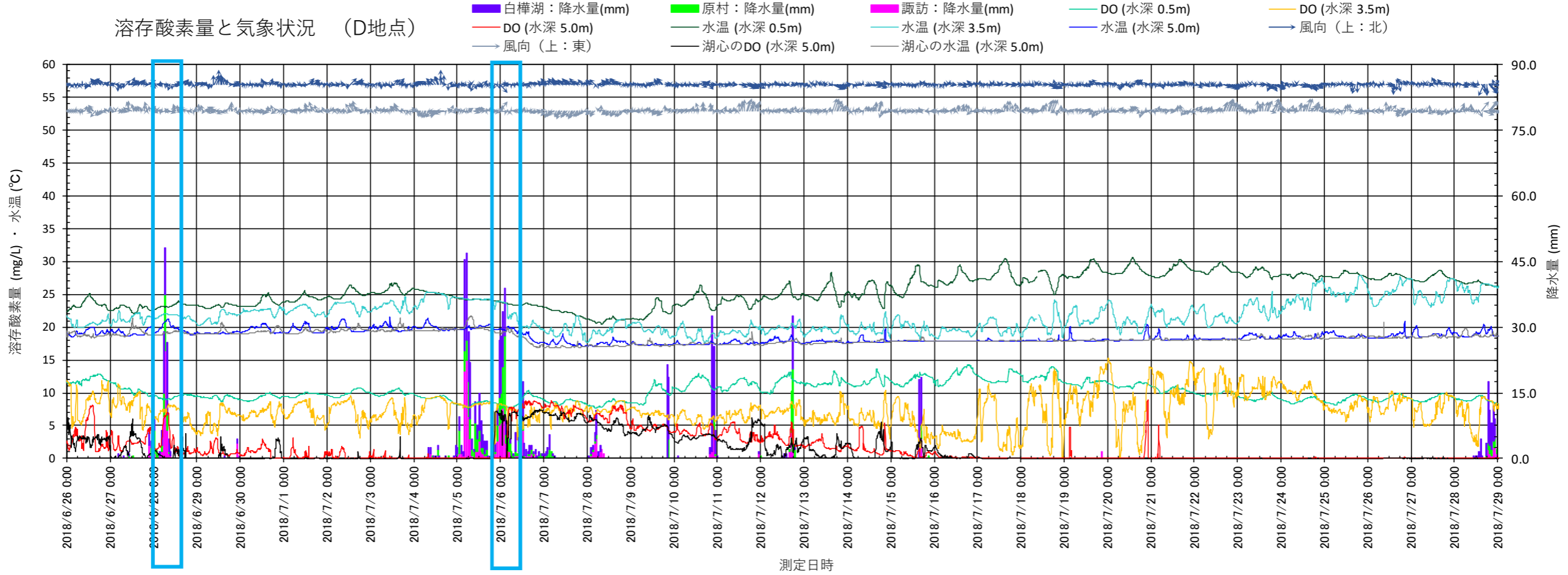
図 3.1.46 (1) 2018 (平成 30) 年度における溶存酸素量と気象状況 (D 地点)
