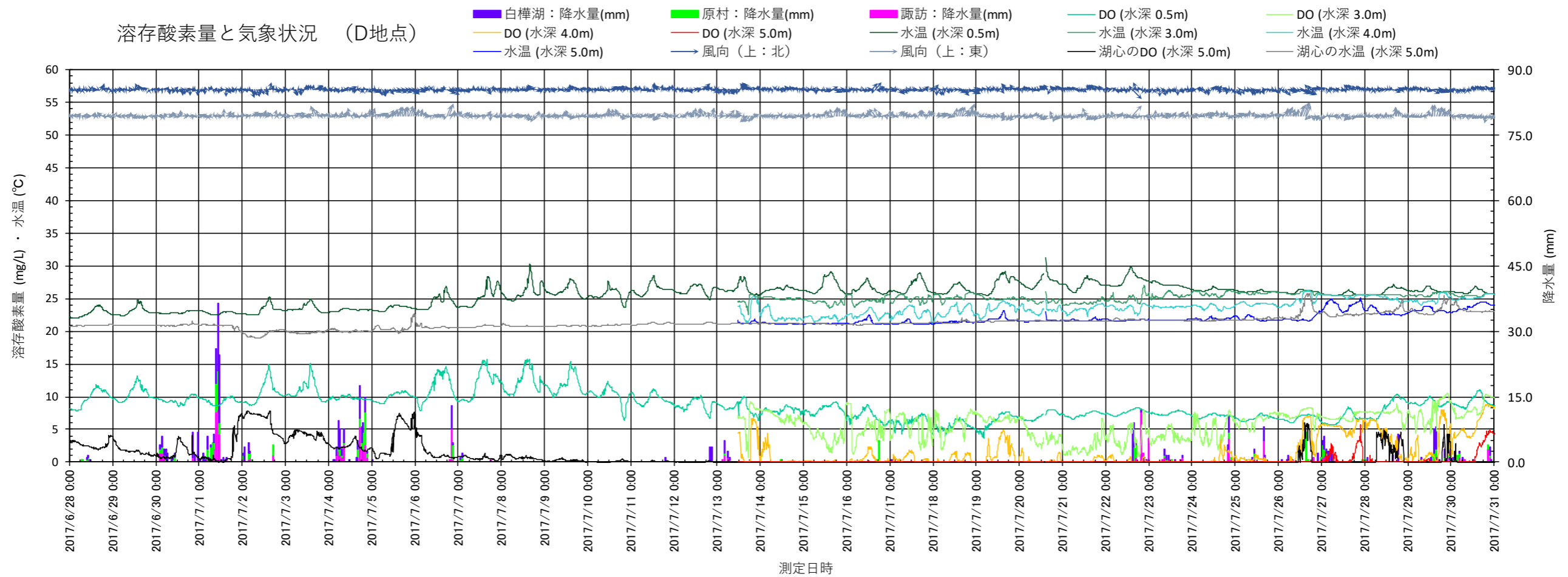
図 3.1.45 (1) 2017 (平成 29) 年度における溶存酸素量と気象状況 (D 地点)
