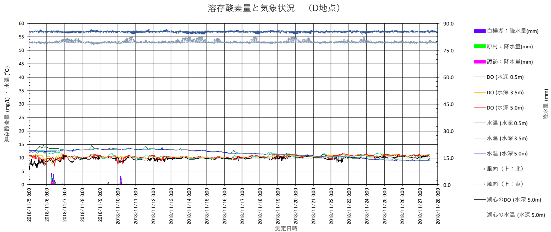
図 3.1.46 (3) 2018 (平成 30) 年度における溶存酸素量と気象状況 (D 地点)
