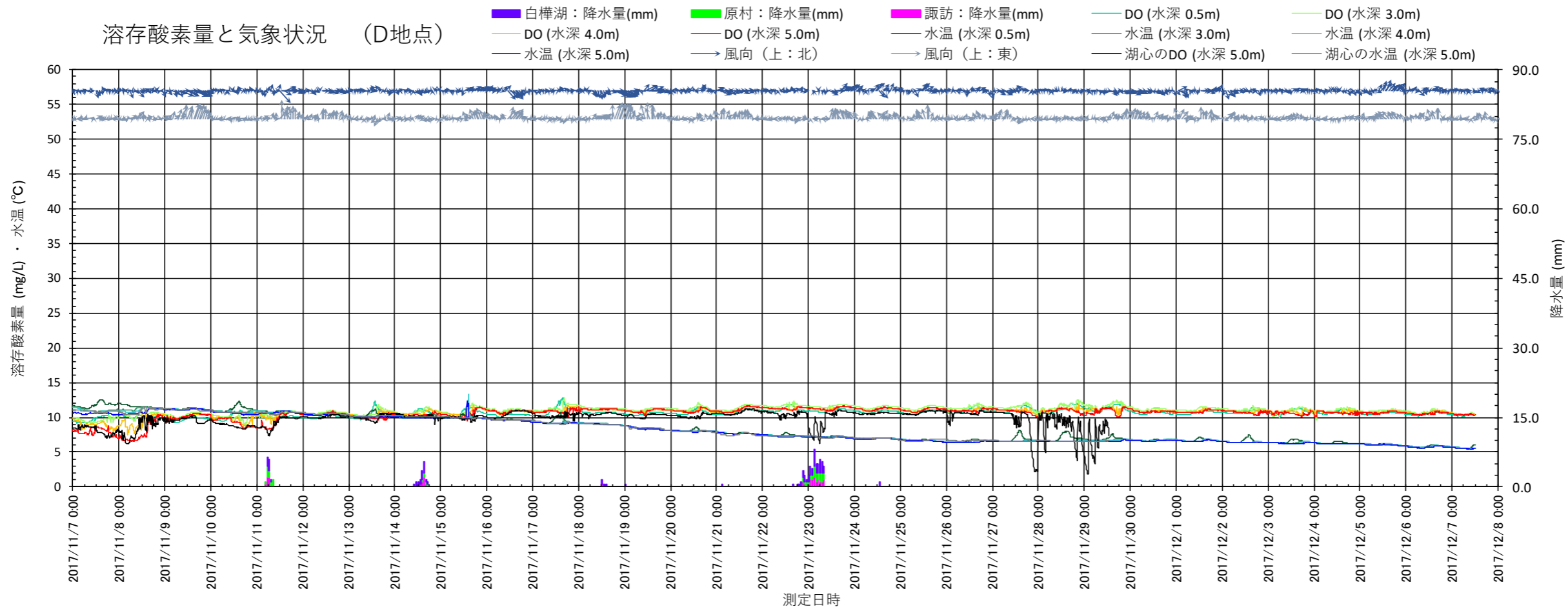
図 3.1.45 (3) 2017 (平成 29) 年度における溶存酸素量と気象状況 (D 地点)
