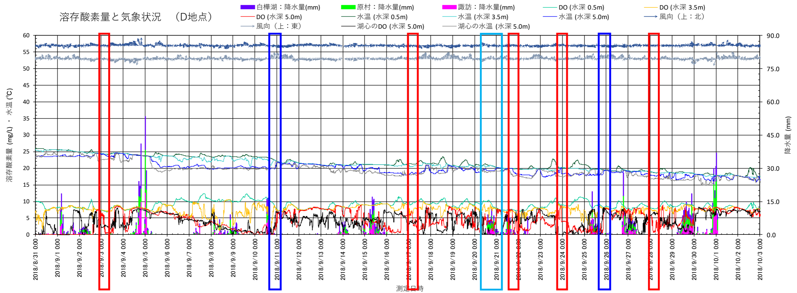
図 3.1.46 (2) 2018 (平成 30) 年度における溶存酸素量と気象状況 (D 地点)
