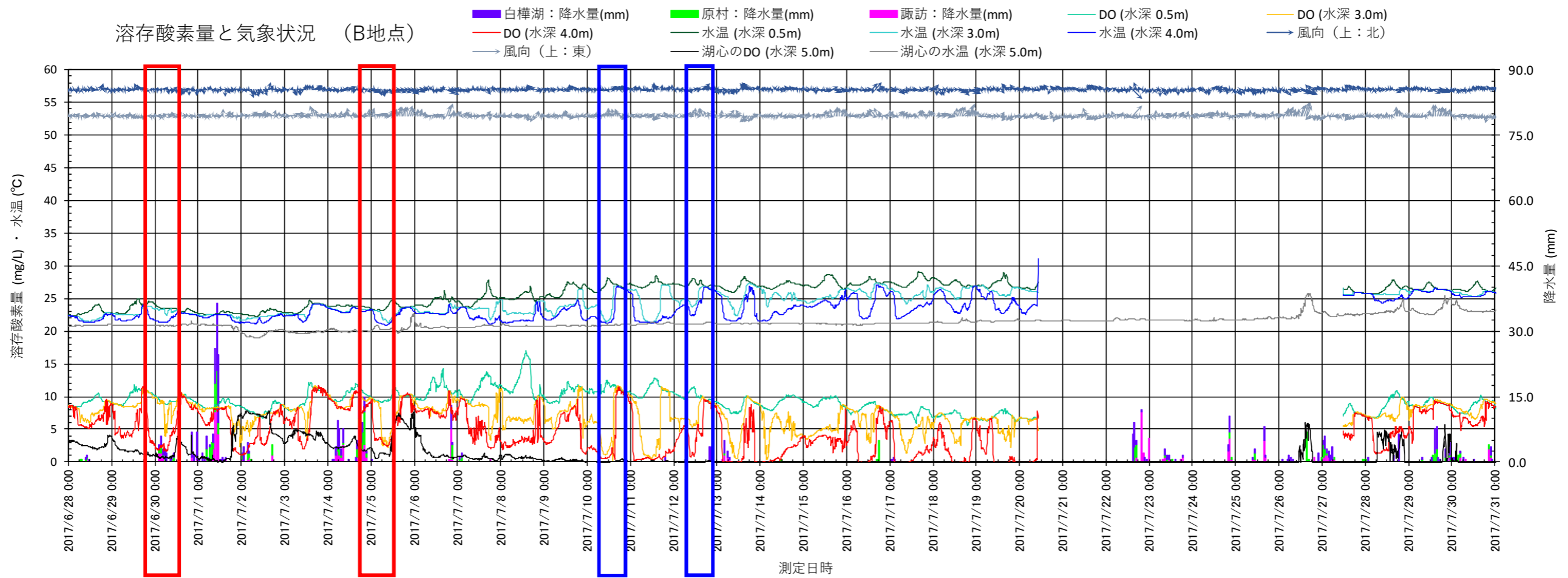
図 3.1.41 (1) 2017 (平成 29) 年度における溶存酸素量と気象状況 (B 地点)
