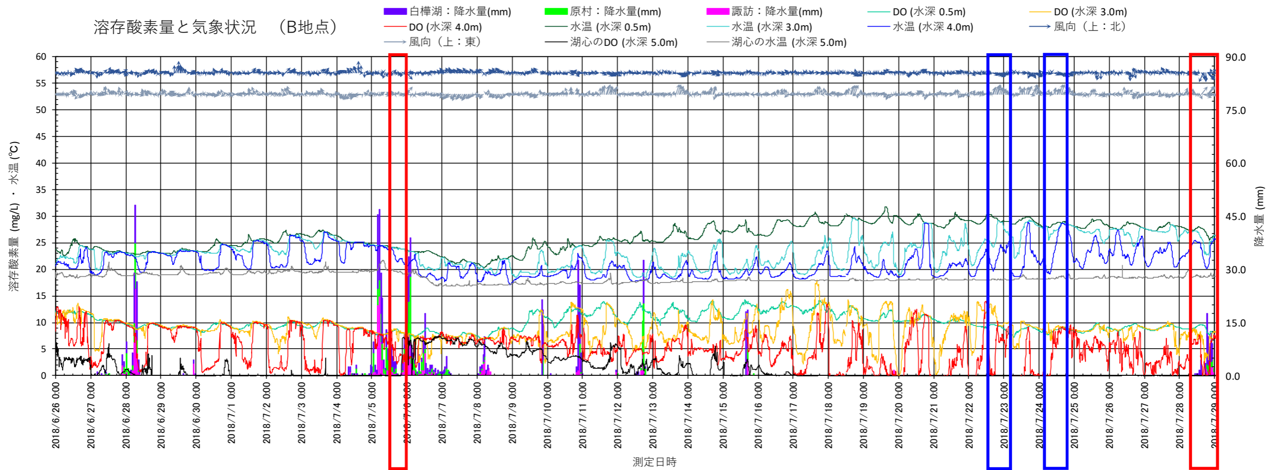
図 3.1.42 (1) 2018 (平成 30) 年度における溶存酸素量と気象状況 (B 地点)
