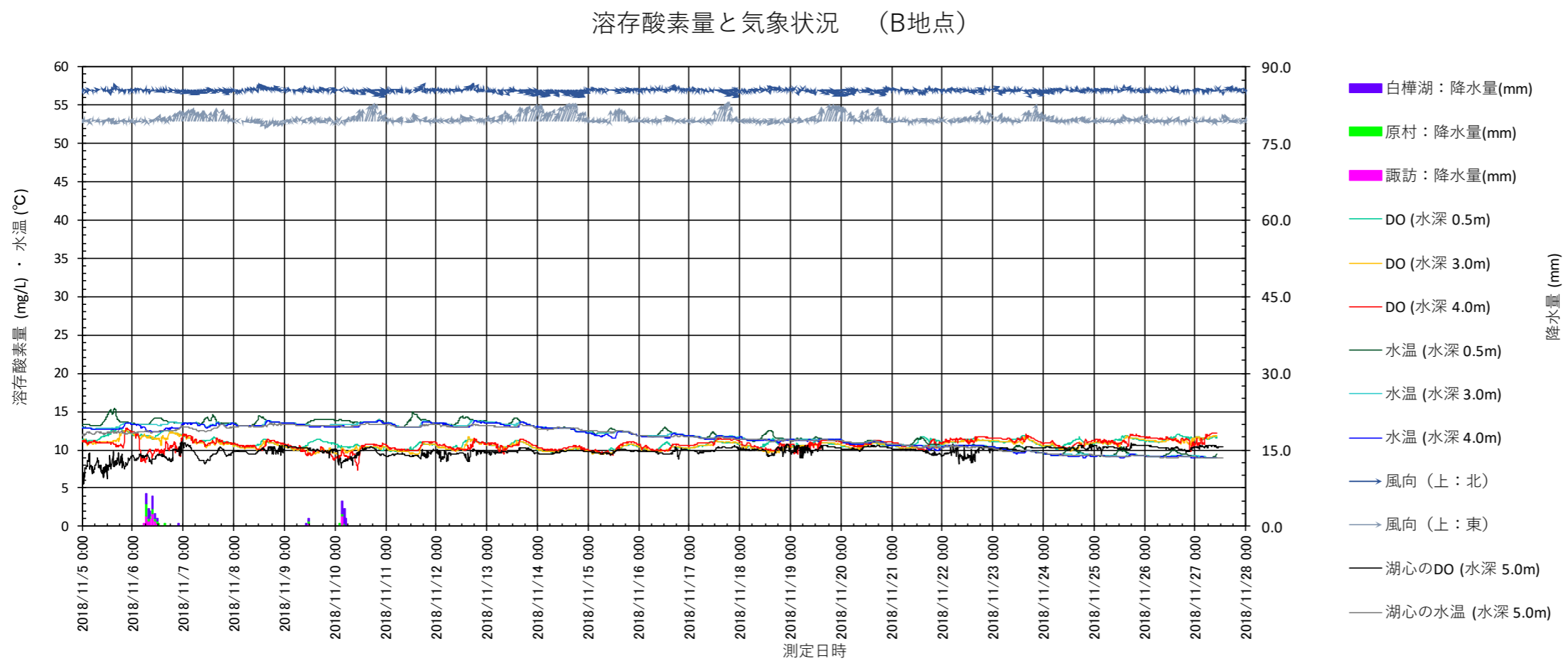
図 3.1.42 (3) 2018 (平成 30) 年度における溶存酸素量と気象状況 (B 地点)
