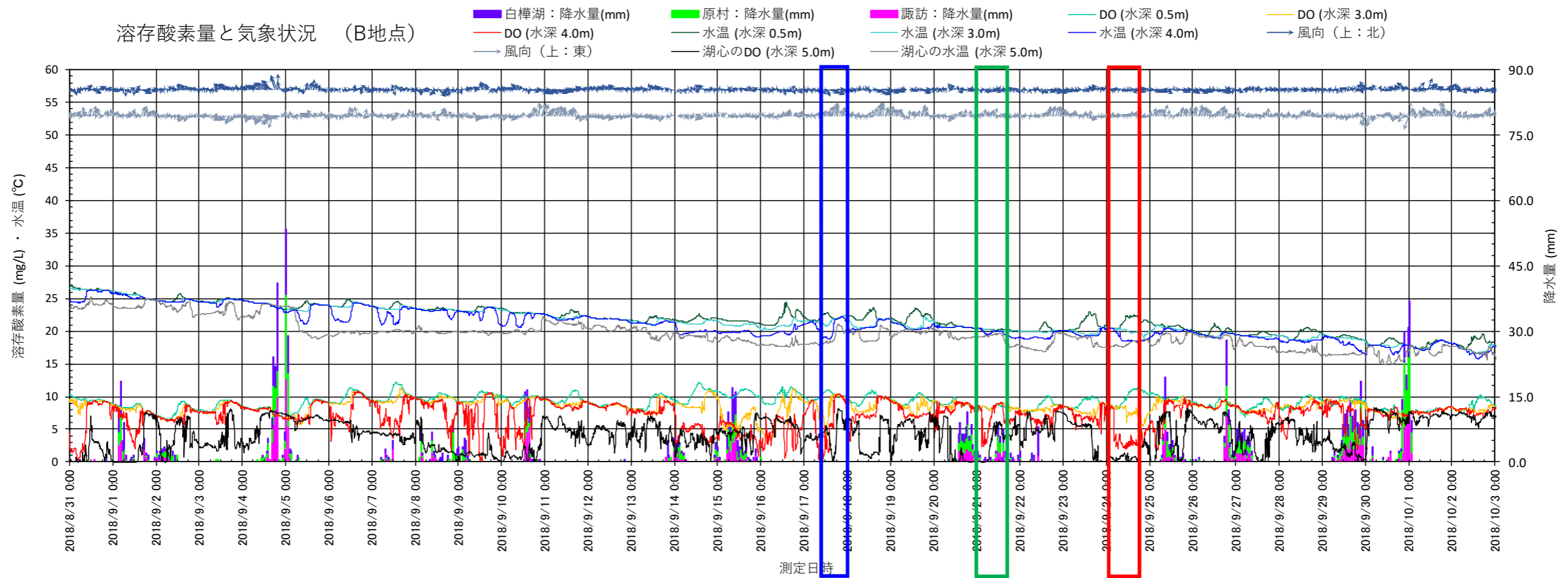
図 3.1.42 (2) 2018 (平成 30) 年度における溶存酸素量と気象状況 (B 地点)
