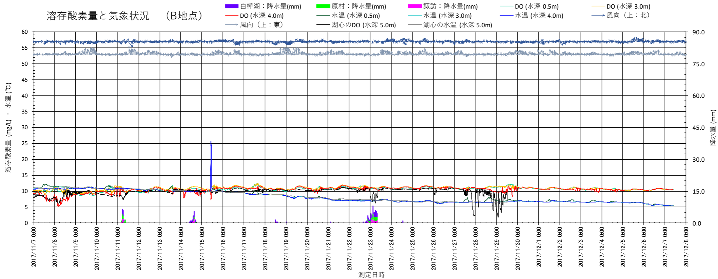
図 3.1.41 (3) 2017 (平成 29) 年度における溶存酸素量と気象状況 (B 地点)
