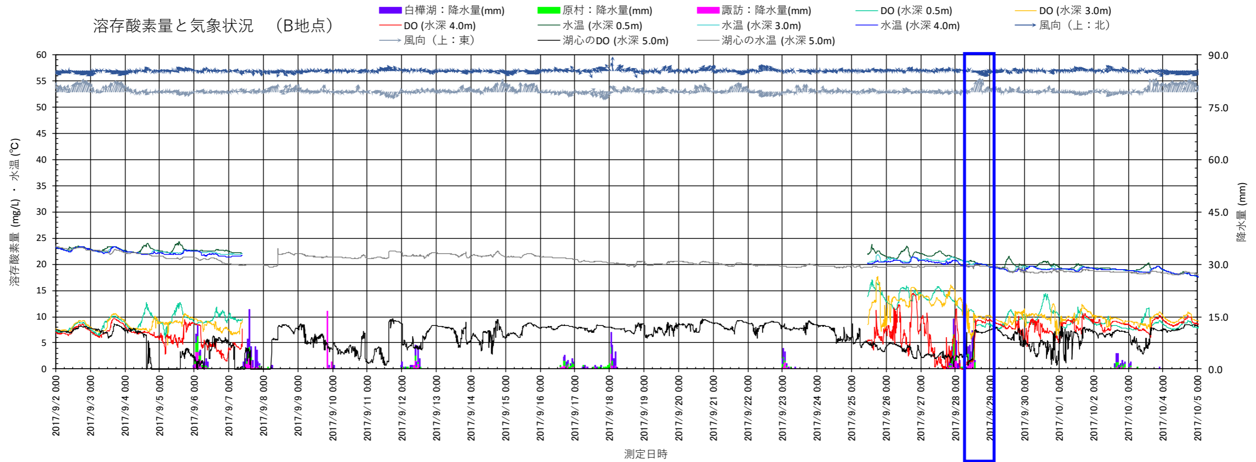
図 3.1.41 (2) 2017 (平成 29) 年度における溶存酸素量と気象状況 (B 地点)
