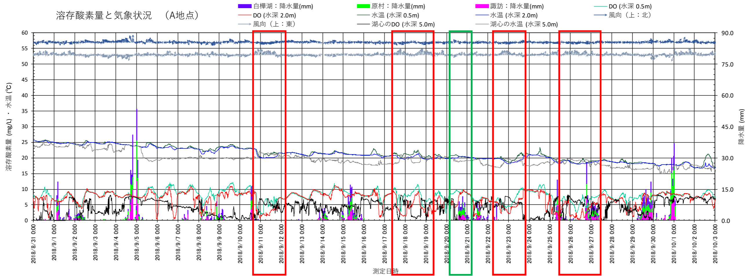
図 3.1.40 (2) 2018 (平成 30) 年度における溶存酸素量と気象状況 (A 地点)
