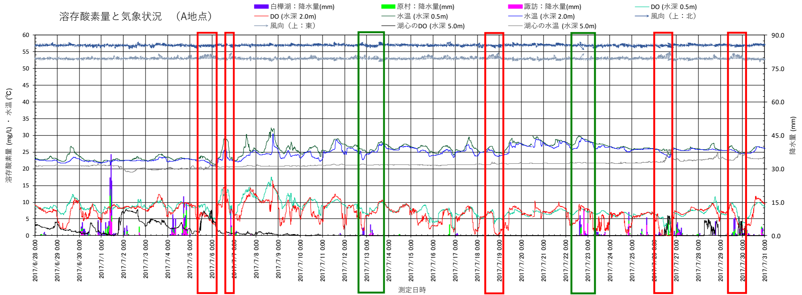
図 3.1.39 (1) 2017 (平成 29) 年度における溶存酸素量と気象状況 (A 地点)
