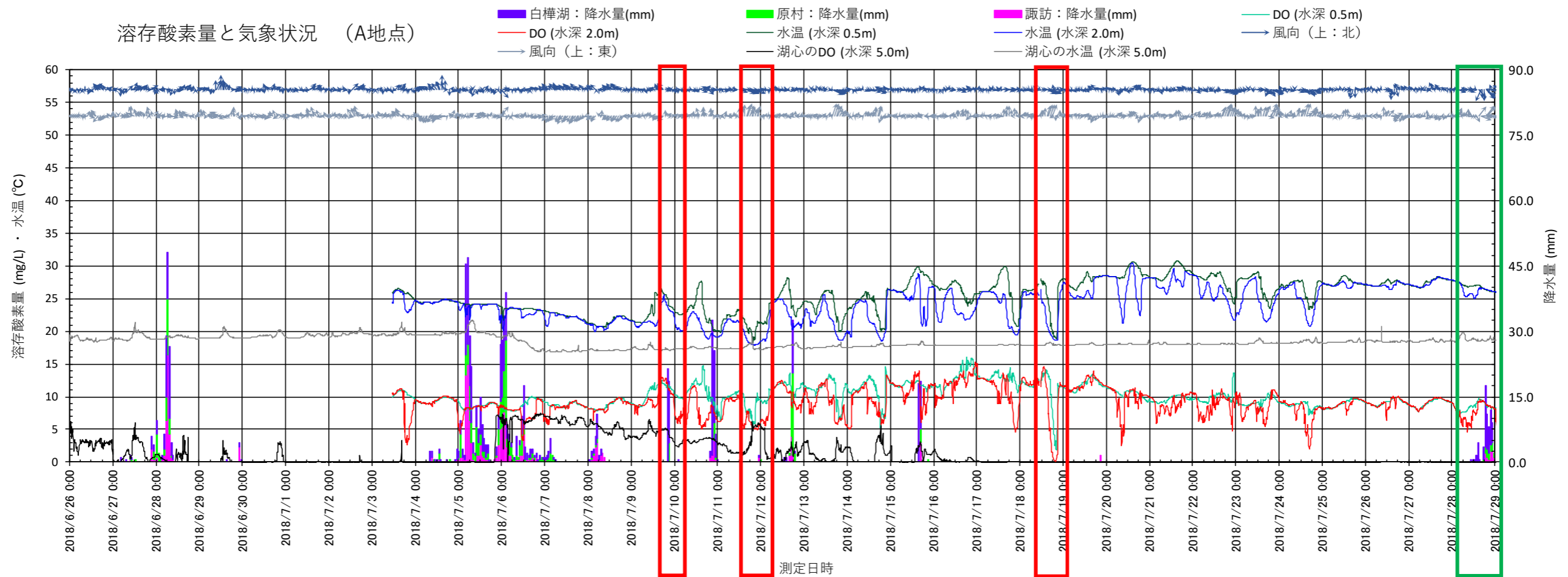
図 3.1.40 (1) 2018 (平成 30) 年度における溶存酸素量と気象状況 (A 地点)
