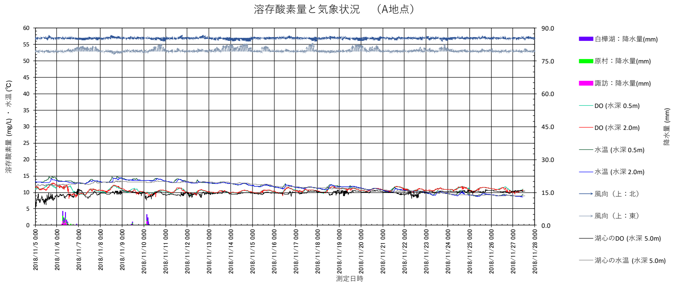
図 3.1.40 (3) 2018 (平成 30) 年度における溶存酸素量と気象状況 (A 地点)
