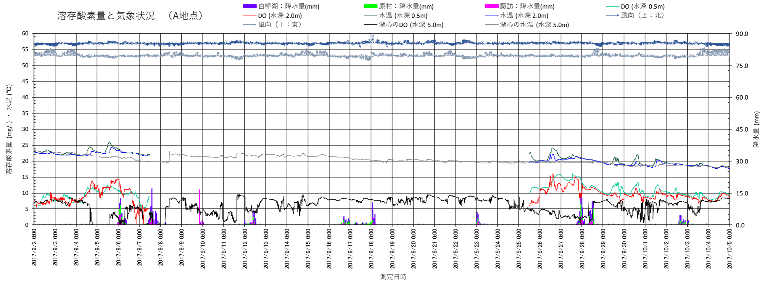
図 3.1.39 (2) 2017 (平成 29) 年度における溶存酸素量と気象状況 (A 地点)
