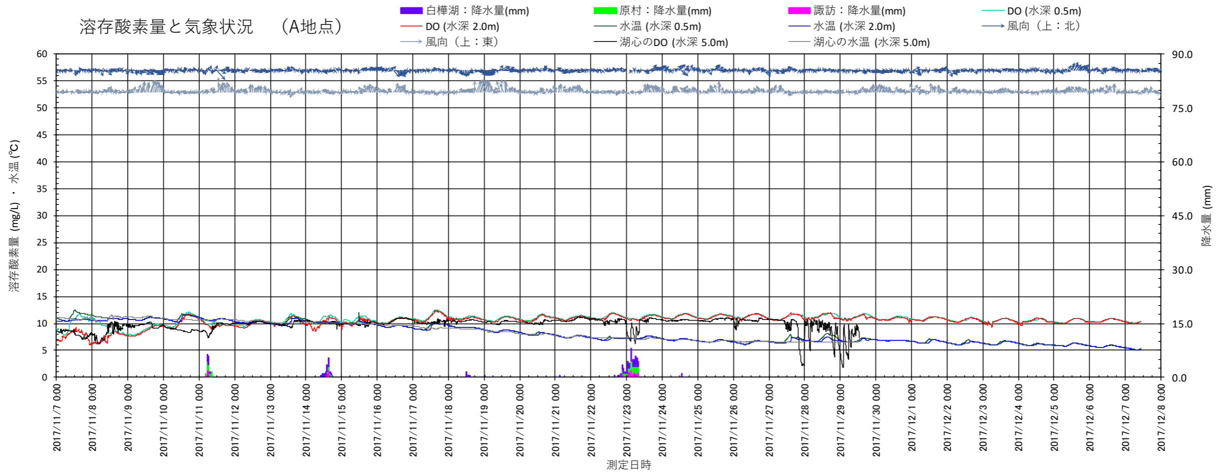
図 3.1.39 (3) 2017 (平成 29) 年度における溶存酸素量と気象状況 (A 地点)
