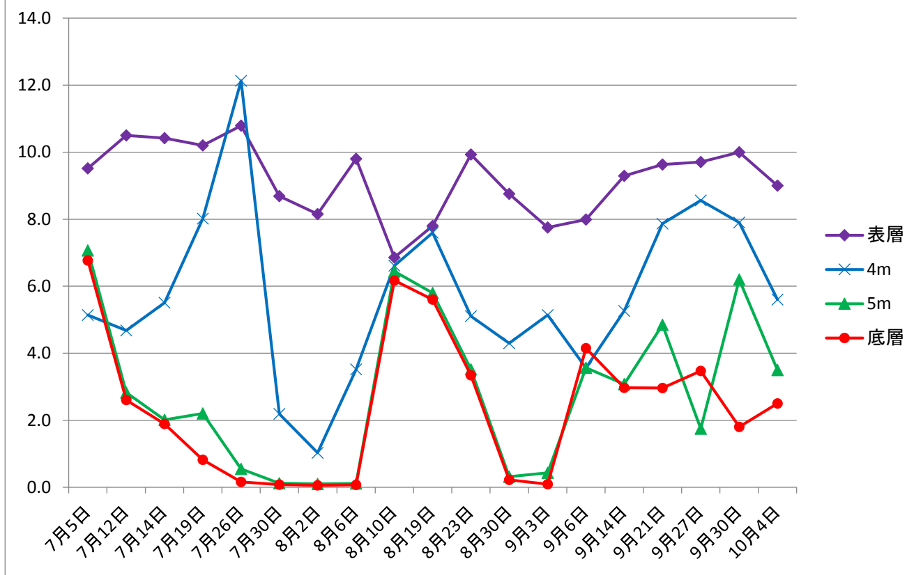
湖心の表層・底層溶存酸素濃度 (mg/L):令和3年度
