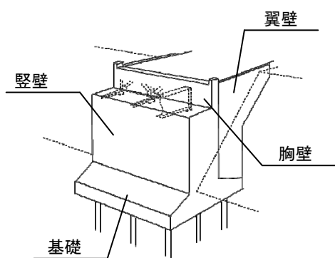
橋台
