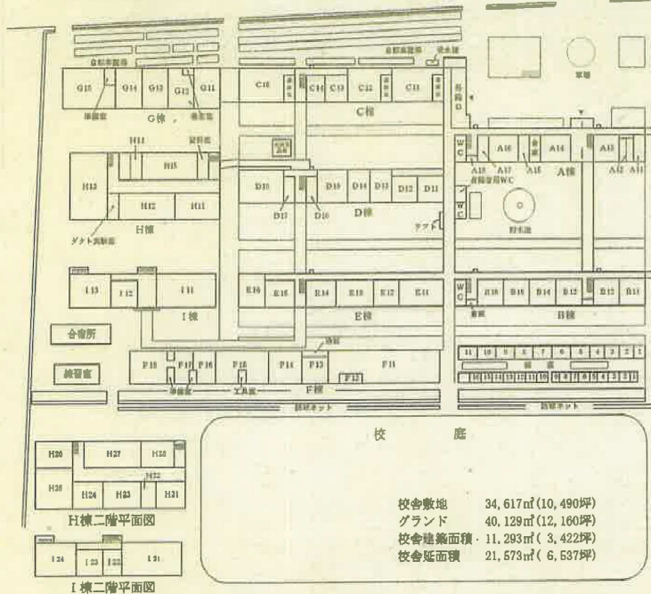
(8) 校舎配置図
