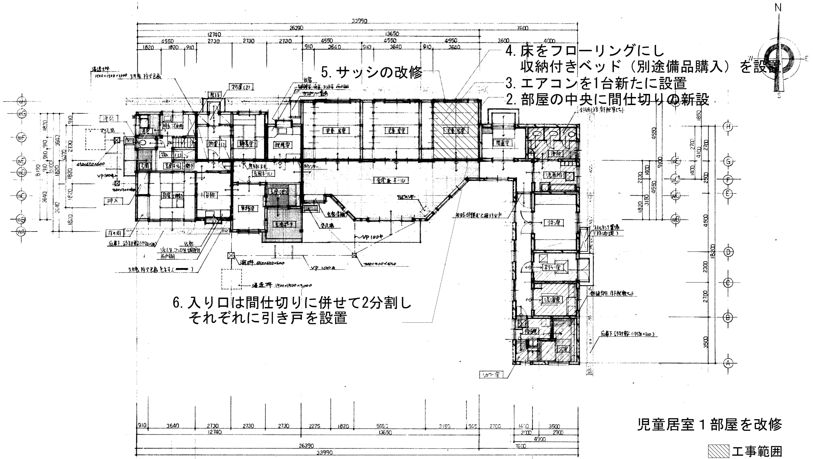
女子寮 平面図
