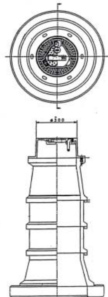
中置弁構造図
