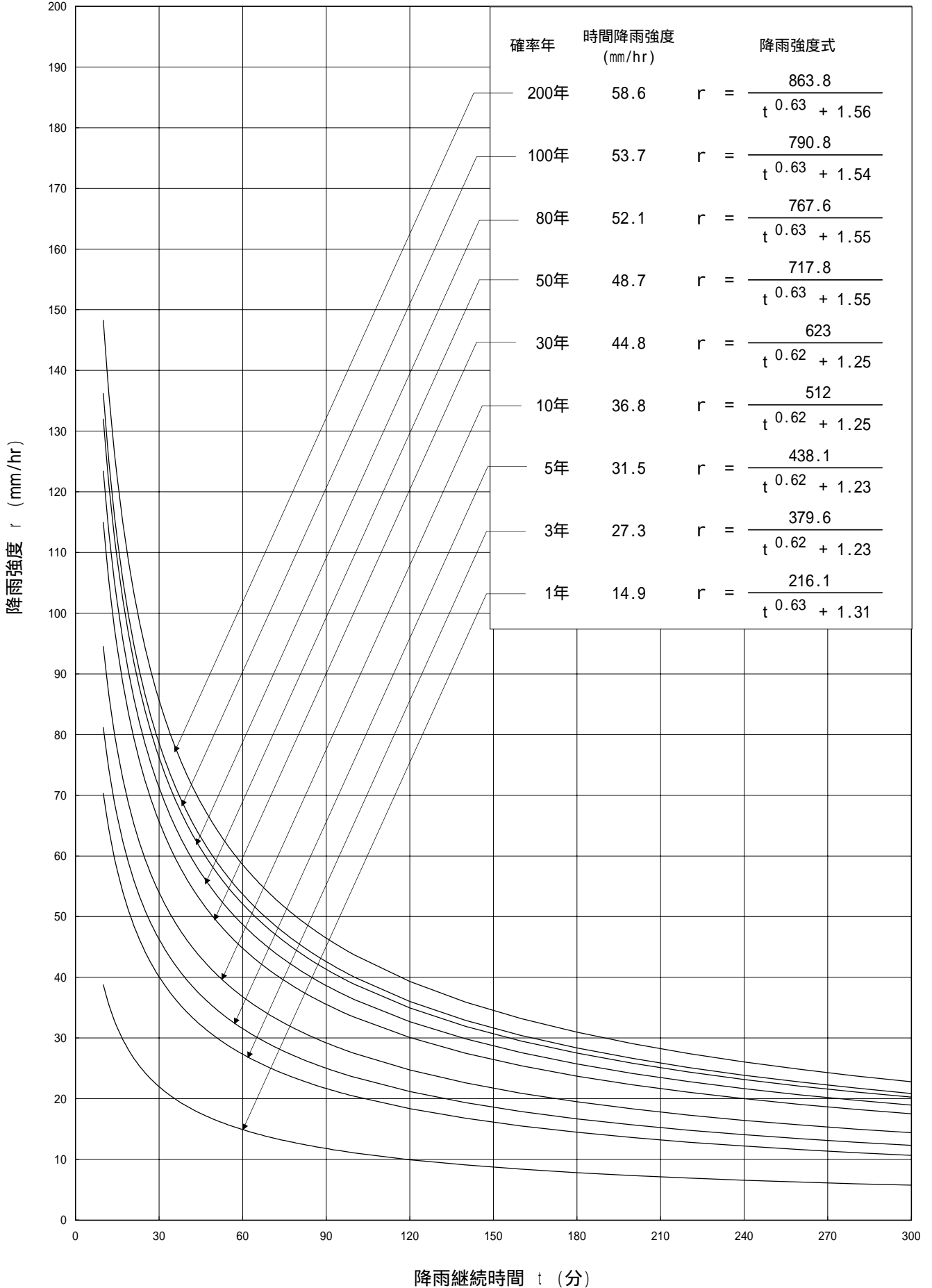
再現年別の降雨強度式と降雨強度曲線 (南佐久領域)
