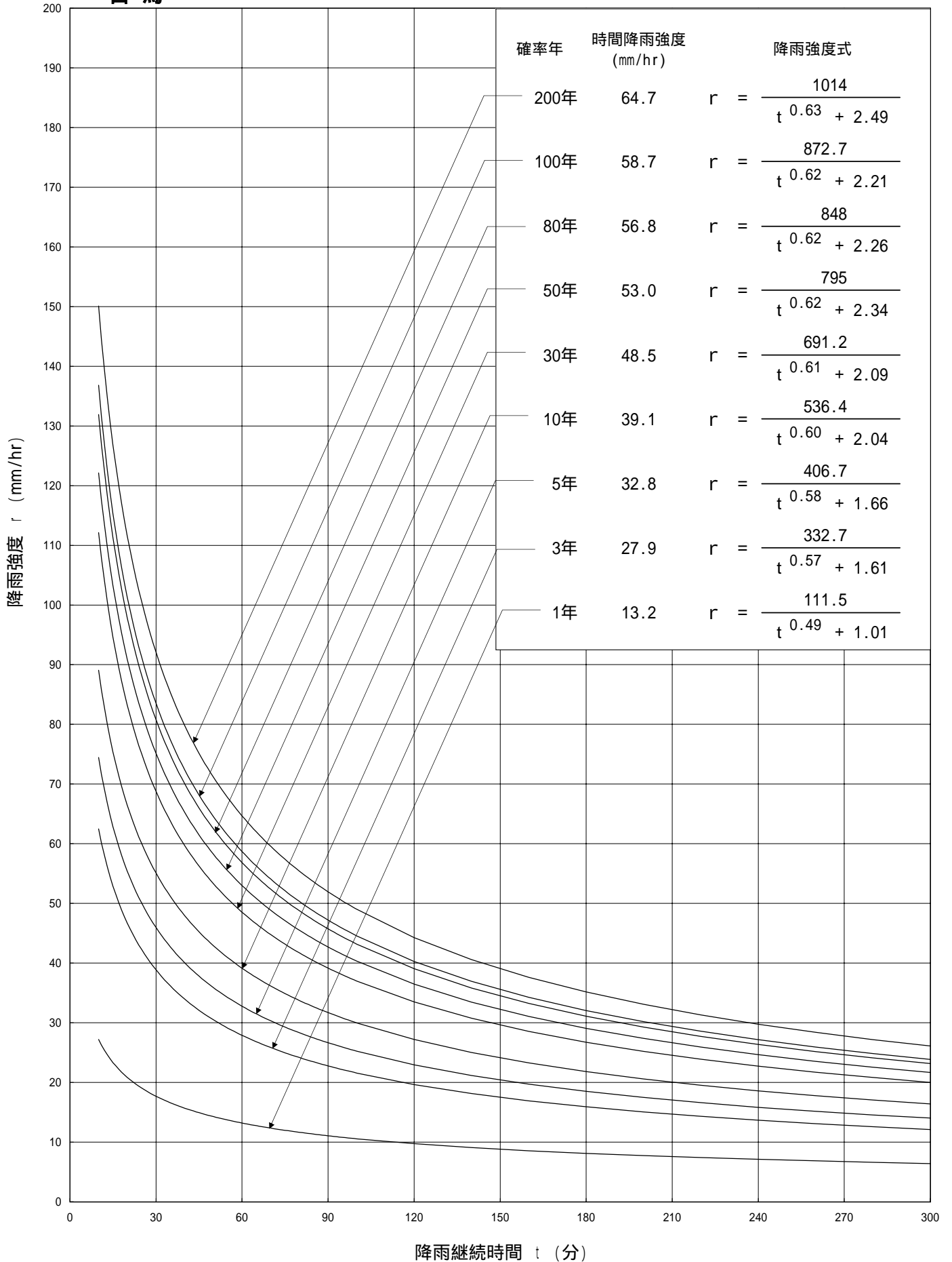
再現年別の降雨強度式と降雨強度曲線 (白馬領域)
