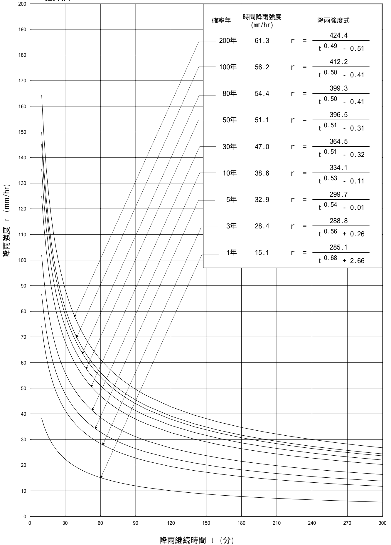
再現年別の降雨強度式と降雨強度曲線 (軽井沢領域)
