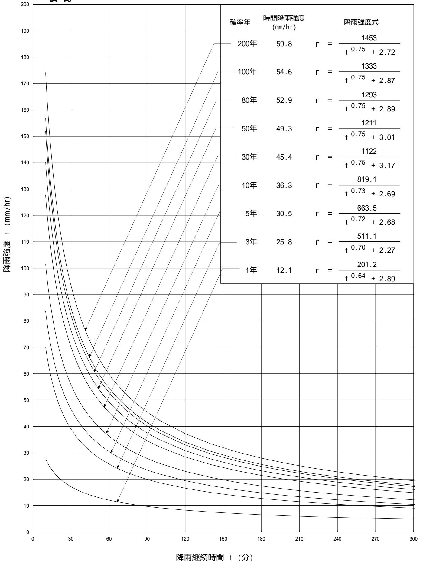
再現年別の降雨強度式と降雨強度曲線 (長野領域)
