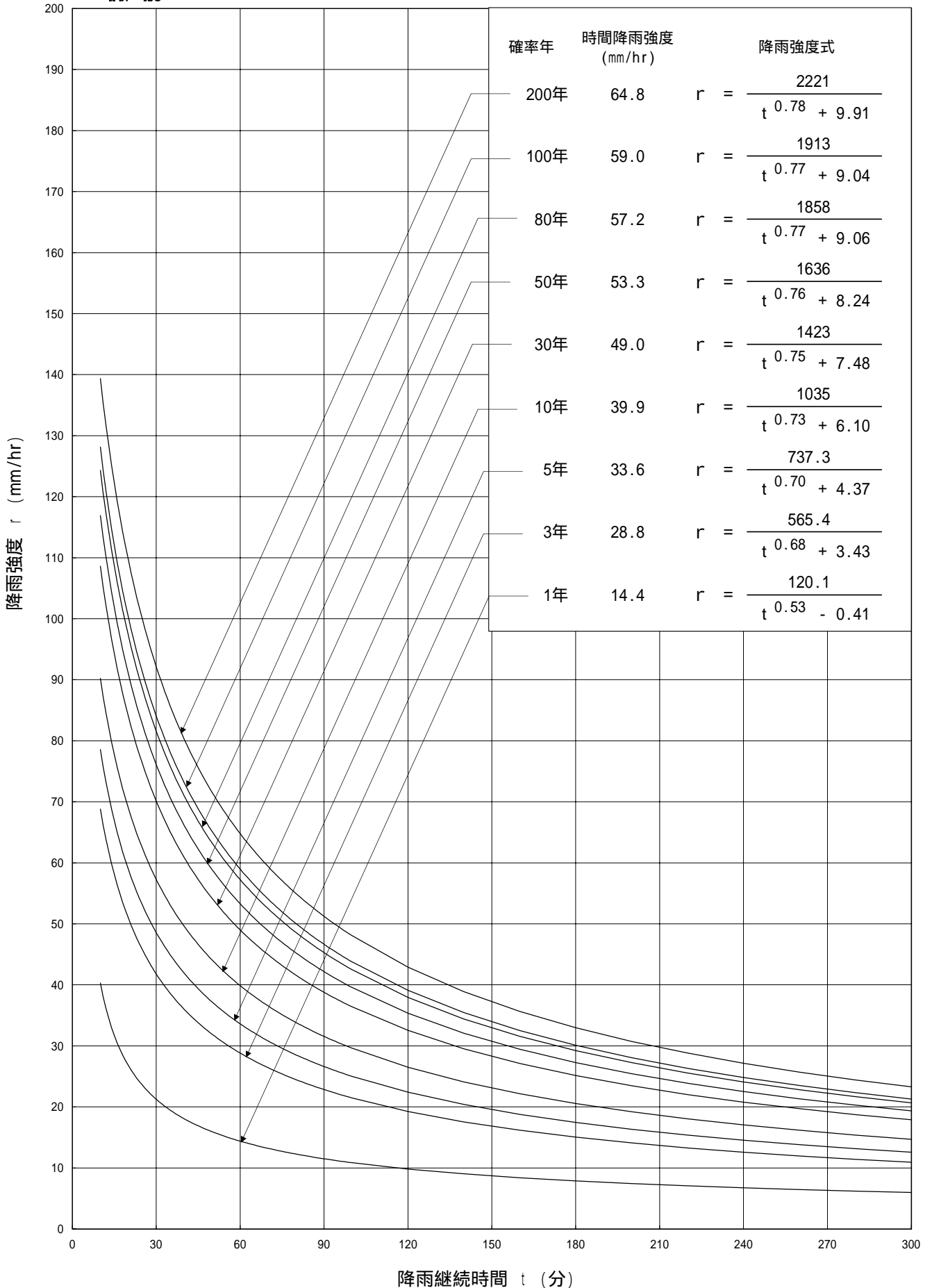
再現年別の降雨強度式と降雨強度曲線 (諏訪領域)
