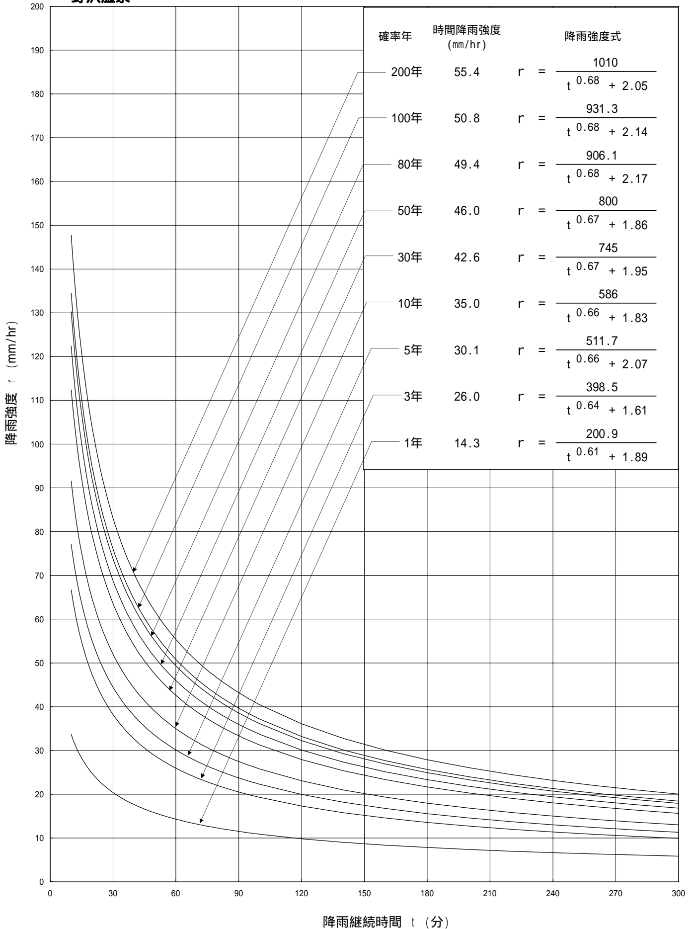
再現年別の降雨強度と降雨強度曲線 (野沢温泉領域)
