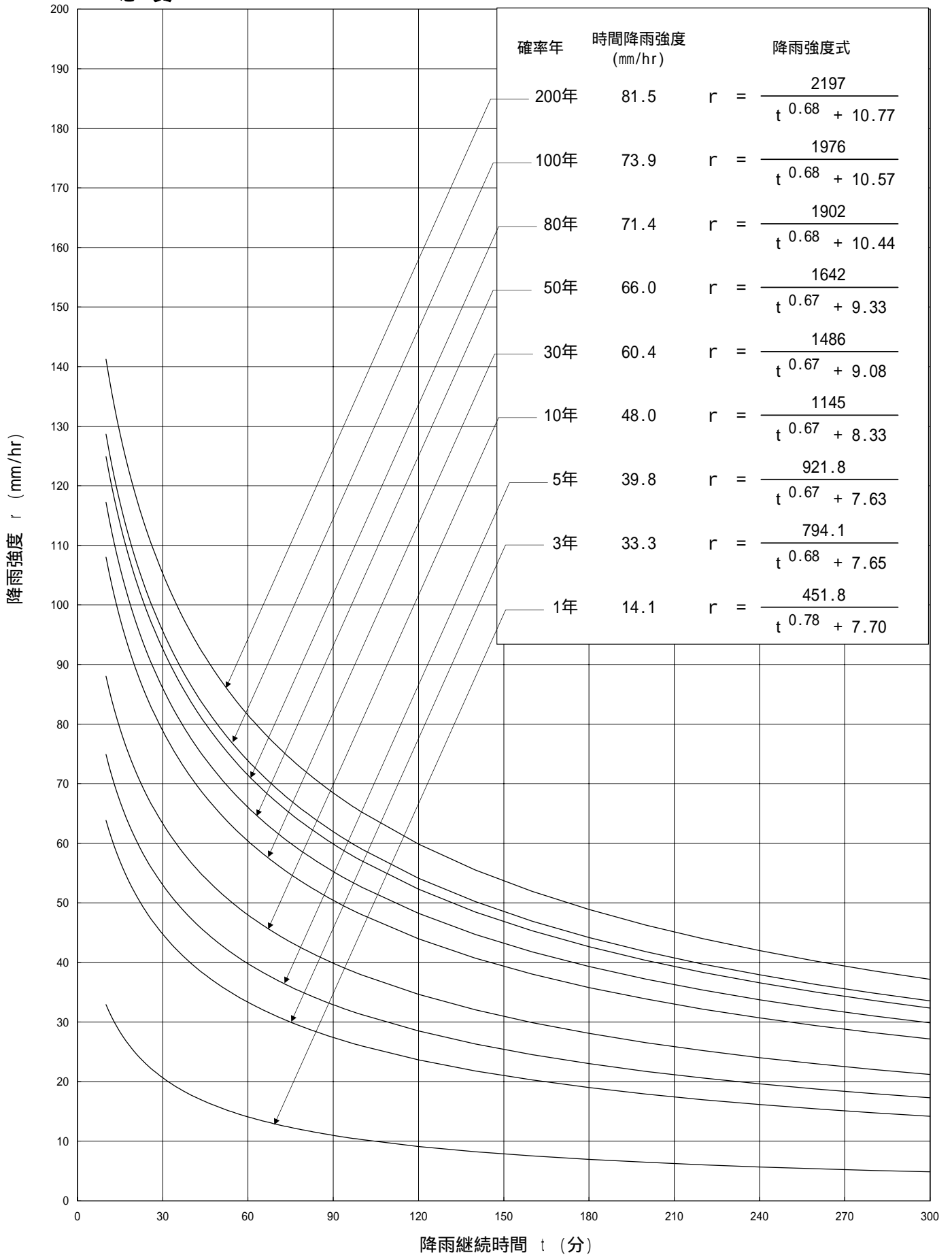
再現年別の降雨強度式と降雨強度曲線 (志賀領域)
