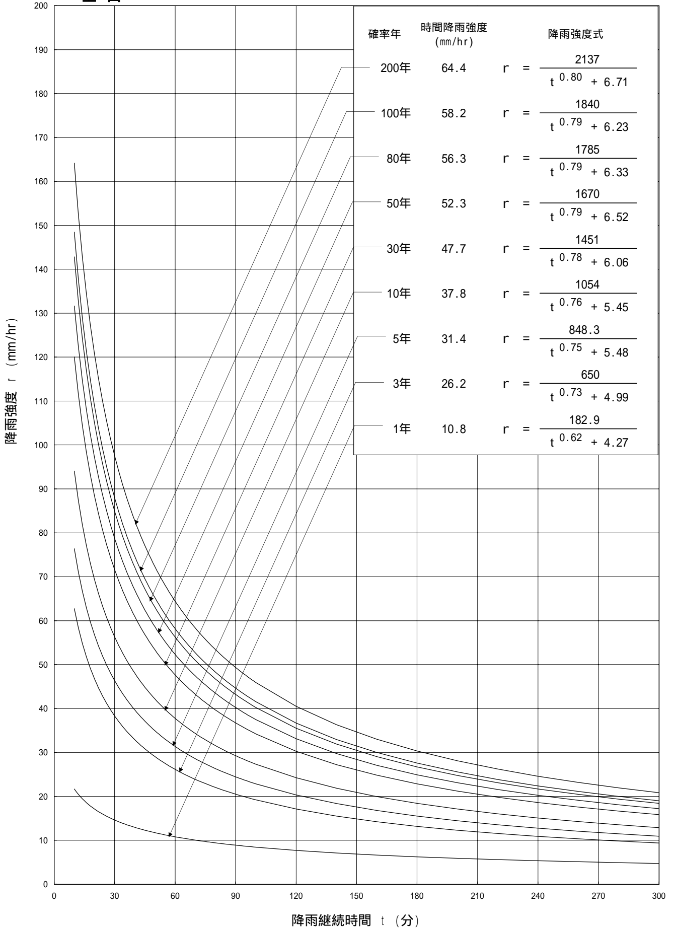
再現年別の降雨強度式と降雨強度曲線 (上田領域)
