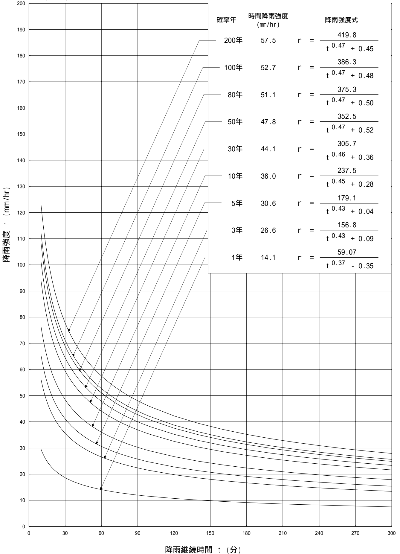
再現年別の降雨強度式と降雨強度曲線 (大町領域)
