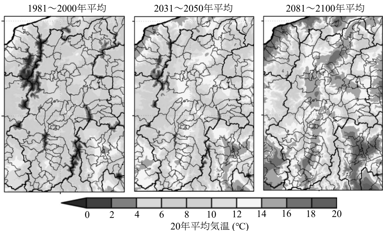
図表2-2-17 N I E S 2020による長野県における年平均気温の将来予測（モデルはMIROC6、シナリオはSSP5-8.5）
