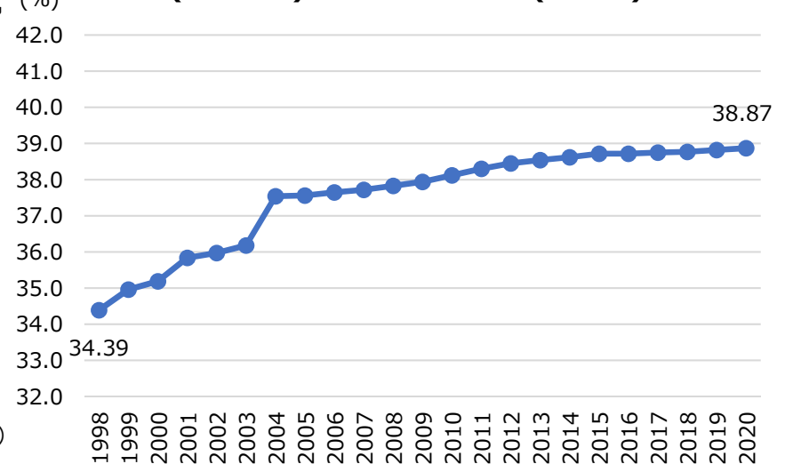
(図7.5-3)河川整備率の推移(長野県)
