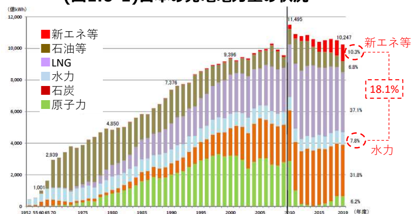
(図1.6-1)日本の発電電力量の状況
