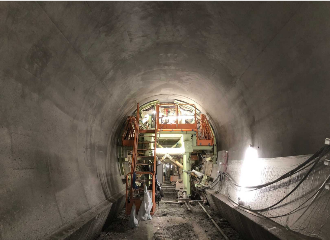
1号トンネル施工状況 (下流より)
