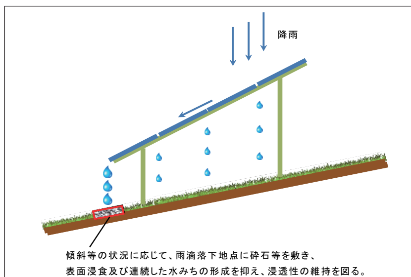
図 4-6-82 太陽光パネル面からの雨滴落下地点の改善措置（概念図）
