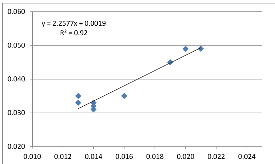
図 2-4-1 日平均値の 2%除外値への変換式 (浮遊粒子状物質)
