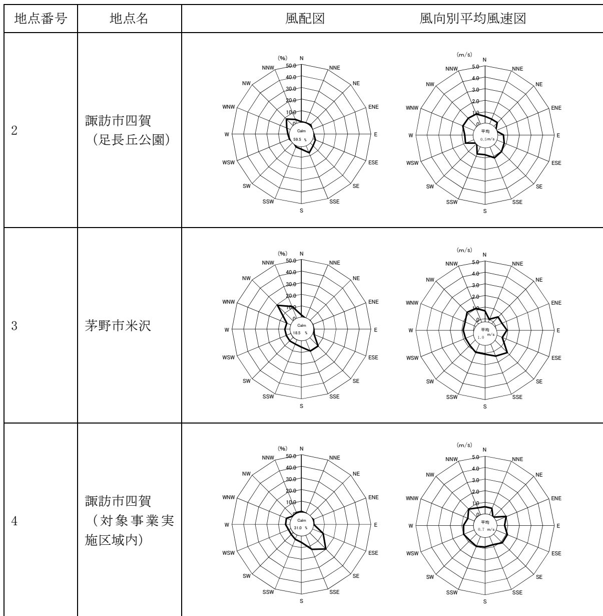
図 4-1-4 風配図 (夏季)
