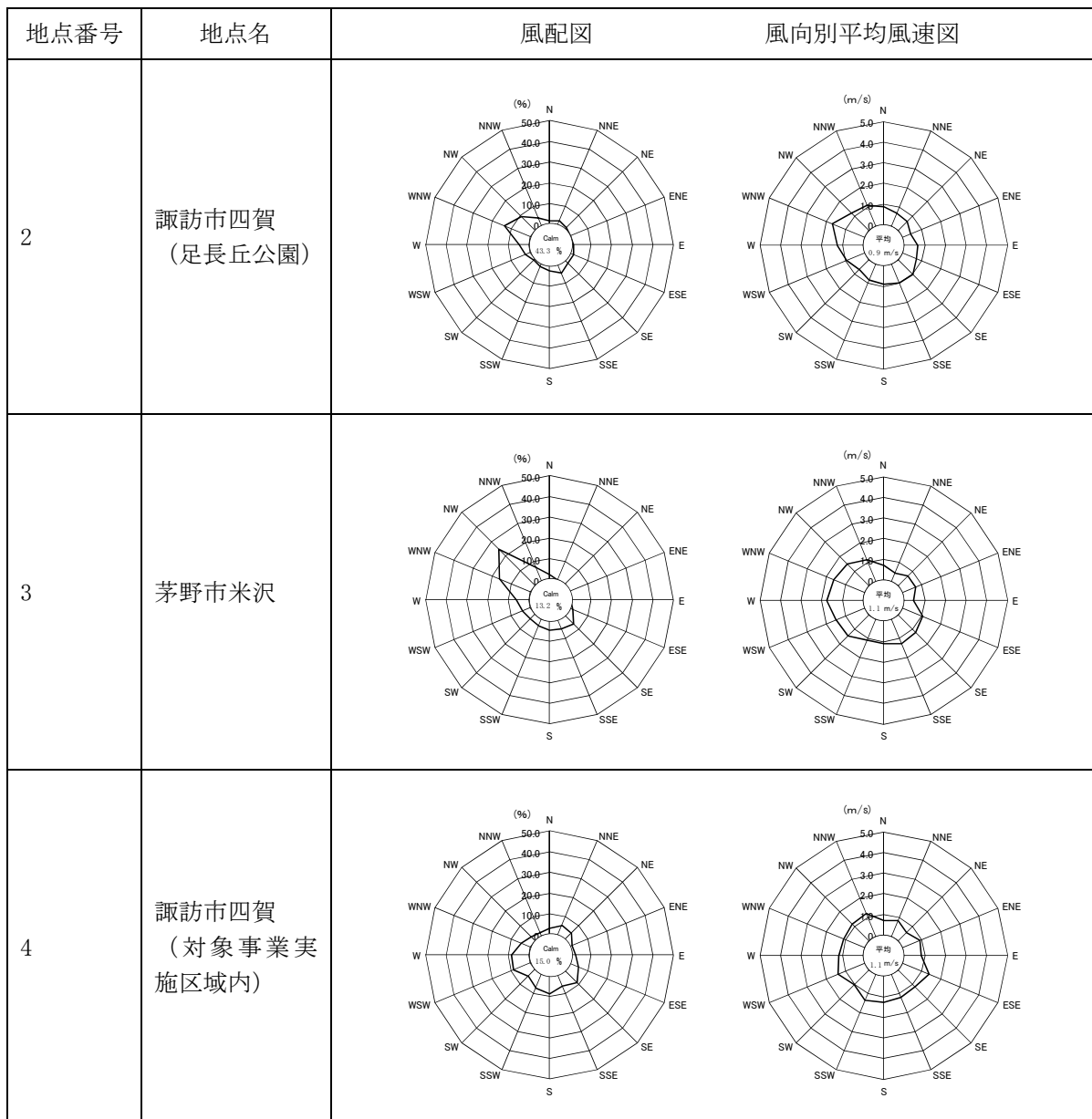
図 4-1-7 風配図 (四季)
