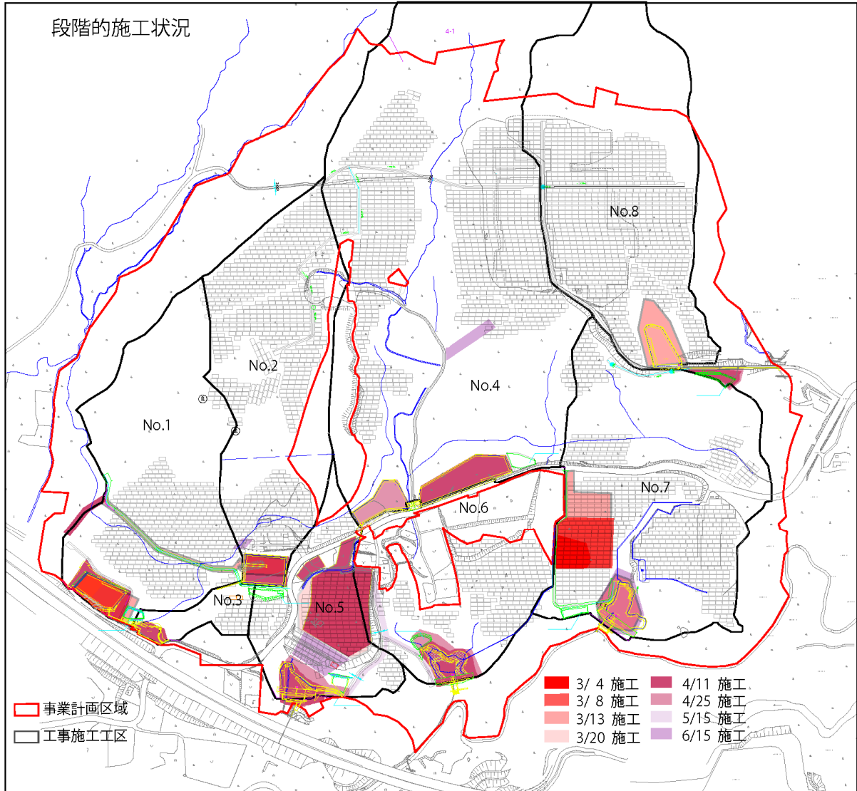
資料4-2：濁水発生抑制に配慮した一時的な広範囲の裸地化抑制による段階的的施工状況
