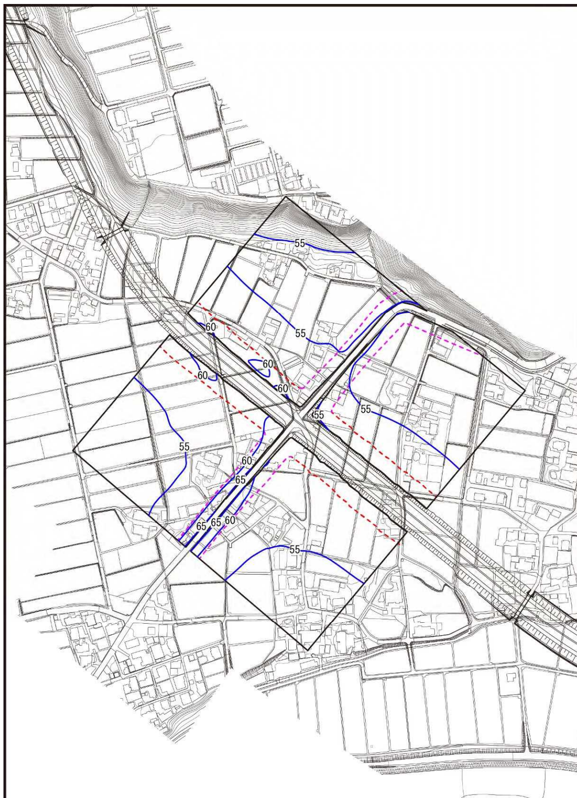
図 3.1-1 (3) 自動車の走行に係る騒音分布図(3. 宮田村大久保)1 階層間
