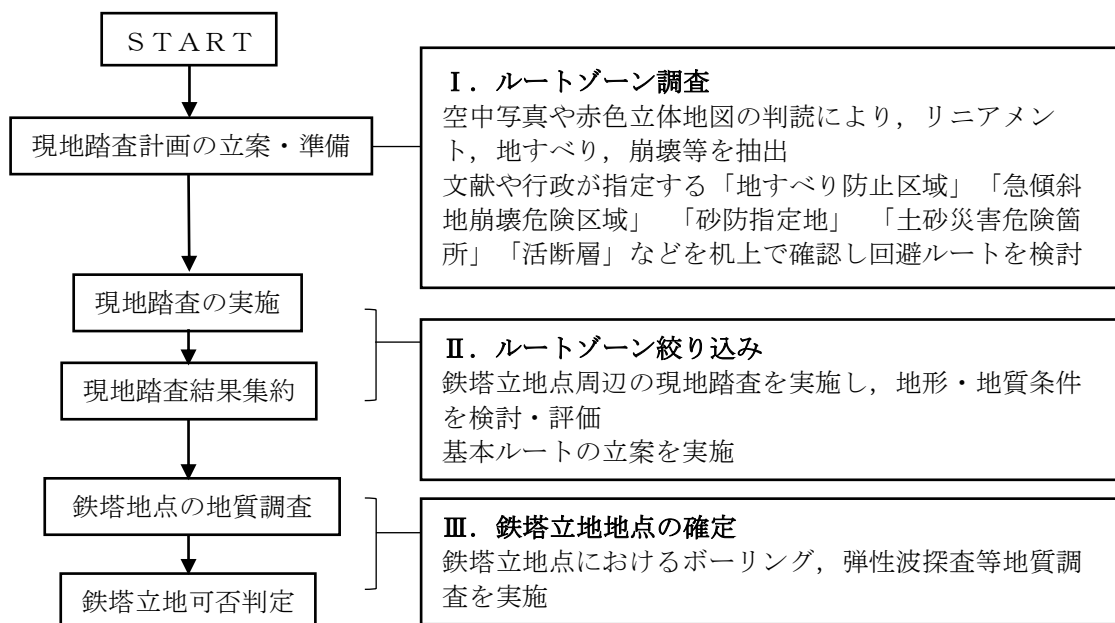
図 5.4-1 鉄塔立地可否判定フロー
