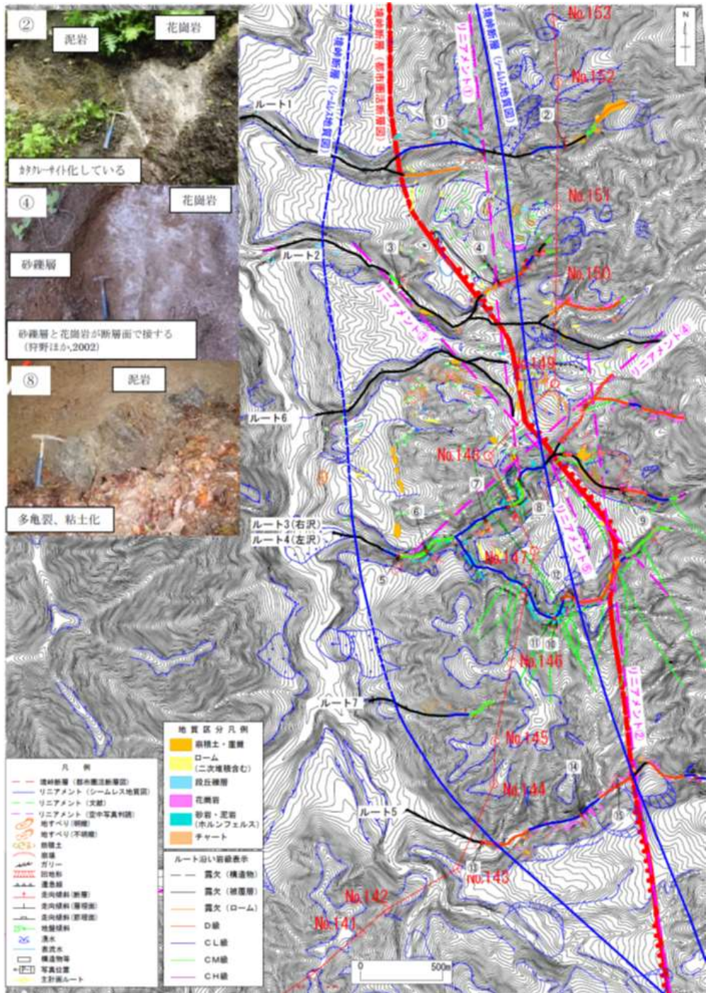
図 5.4-2 境峠断層付近の地形判読・地表踏査結果
