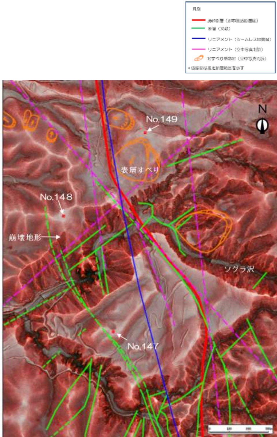
図 5. 4-3 境峠断層と送電線ルート交差位置付近の地形
