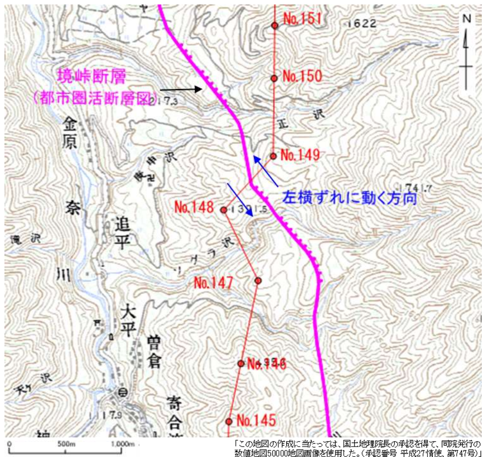
図 5.4-4 境峠断層と送電線ルートの関係
