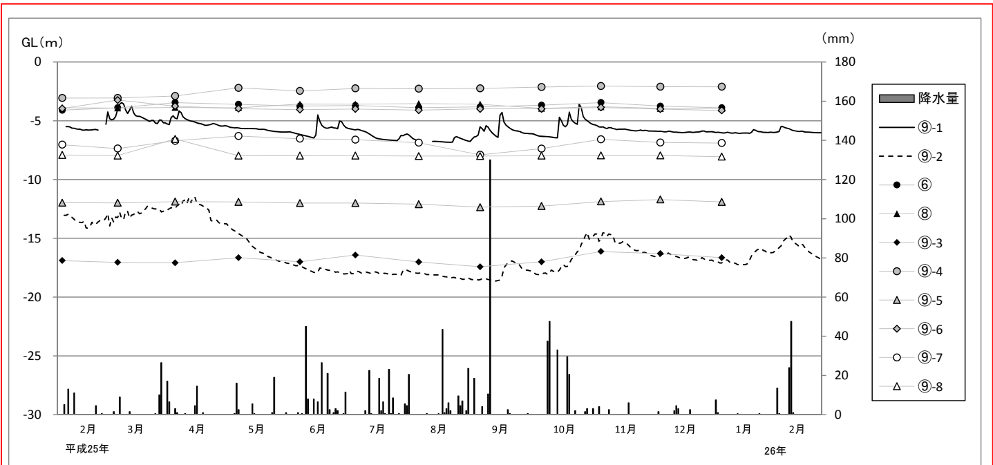
図 地下水位調査結果(1年間連続測定地点)
