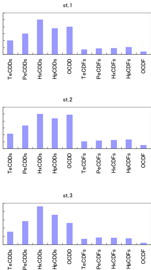
図 II.5.2-2 廃棄物焼却炉の各場所におけるダイオキシン類の同族体パターン
