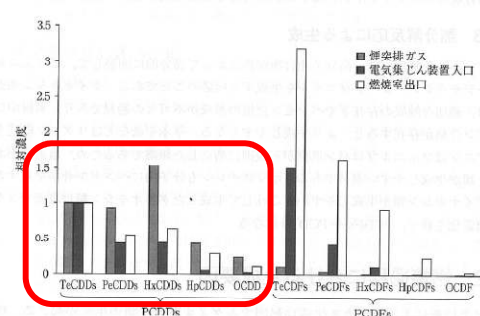
図 II.5.2-2 廃棄物焼却炉の各場所におけるダイオキシン類の同族体パターン
