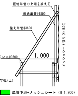
■ 単管下地+メッシュシート (H=1,800)
