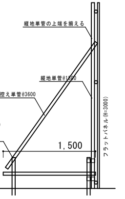
■ フラットパネル (H=3,000)
