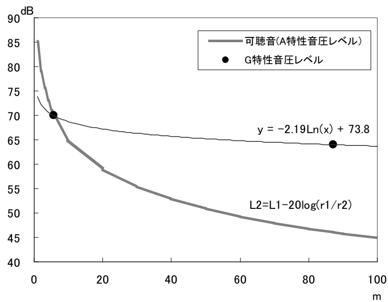
図 4.4-7 低周波音 (G 特性音圧レベル) と可聴音 (A 特性音圧レベル) の距離減衰の比較
