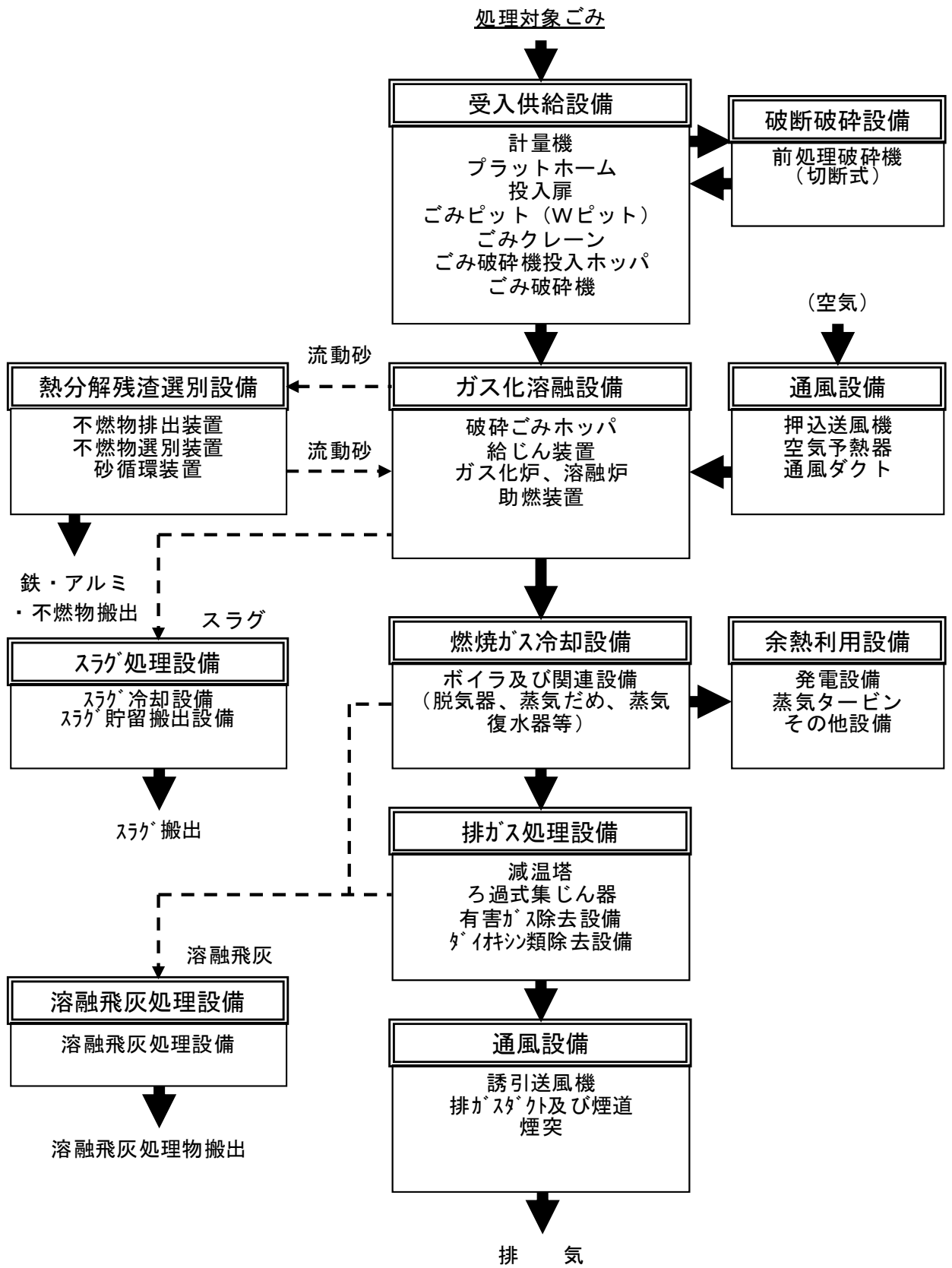
図 1.6-3(1) 処理方式フロー一例 (ガス化溶融方式 (流動床方式))
