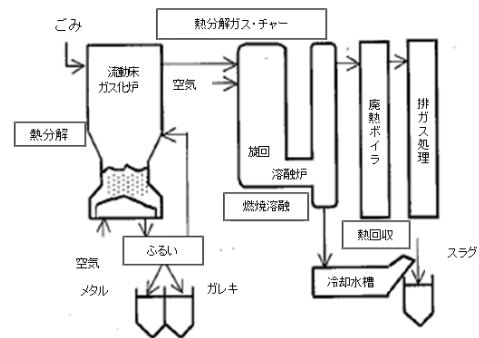
流動床式ガス化溶融方式の概念図
