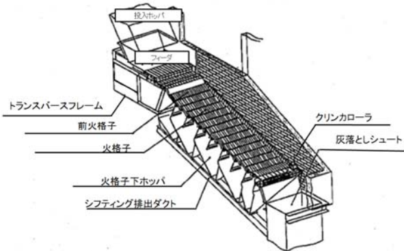
ストーカ式焼却炉の概念図
