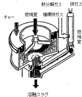
灰溶融（燃料）炉の概念図
