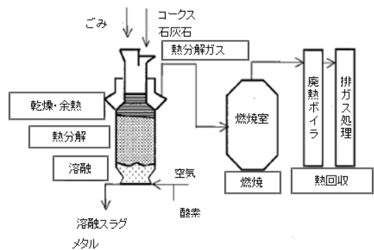
シャフト炉式ガス化溶融炉の概念図
