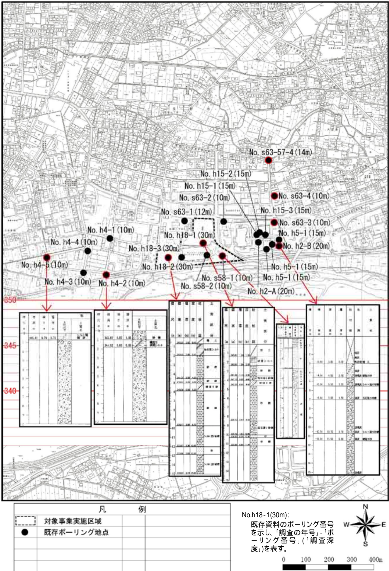
図 4-7-7(1) 対象事業実施区域内及びその周辺におけるボーリング調査結果
