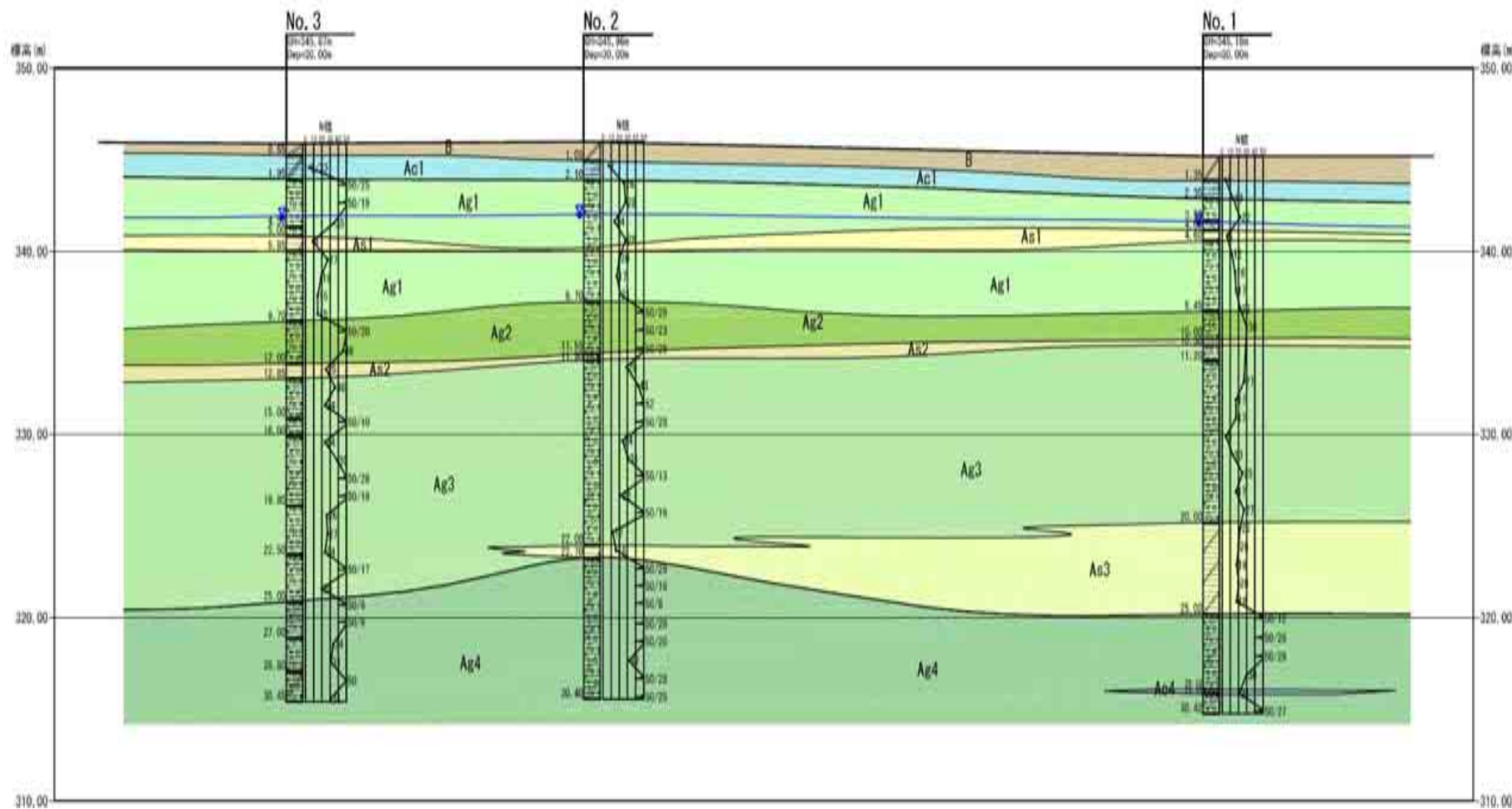
図 4-7-8 対象実施区域の地質断面図
