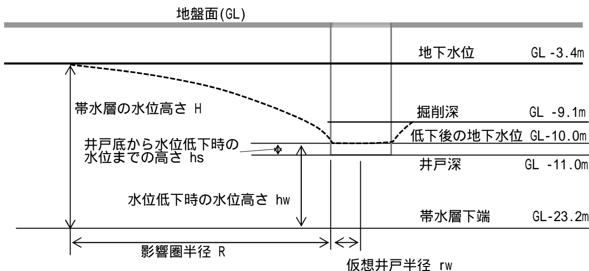
図 4-7-13 検討モデル図
