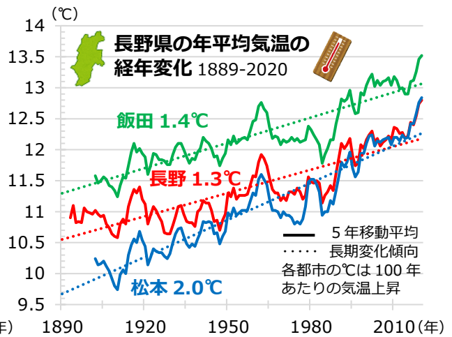
〔出典〕 気象庁データを基に作成
