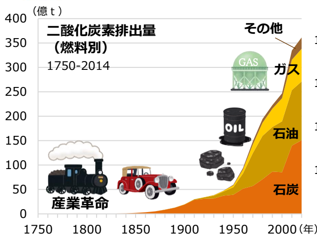
〔出典〕 CDIAC 「Global Fossil-Fuel Carbon Emissions」 他より作成
