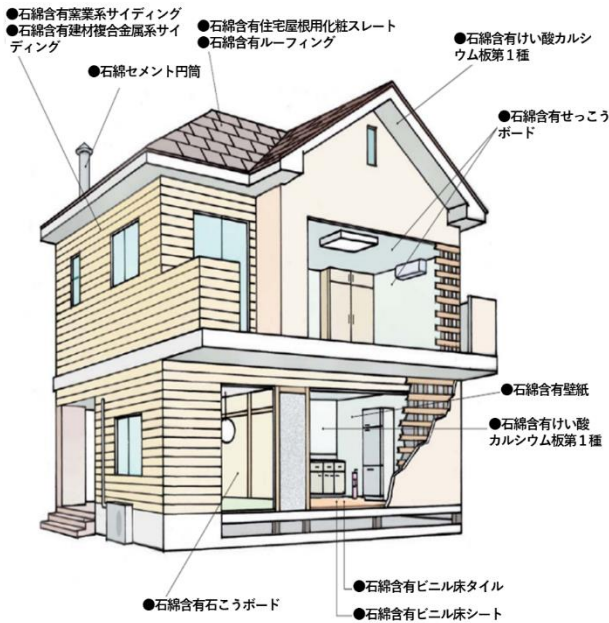
アスベスト含有建材の使用部位(戸建て住宅の例)
