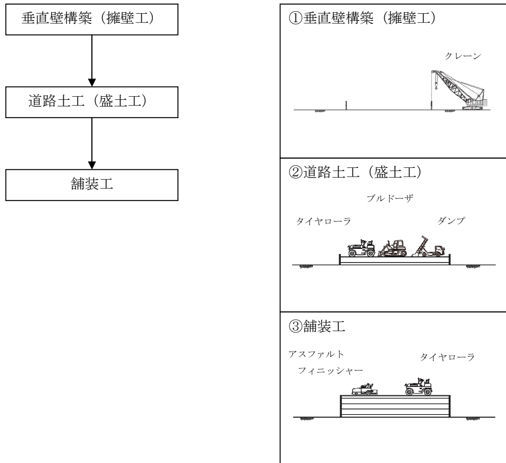
図 3.2.13-3 土工工事(直壁部)の施工順序
