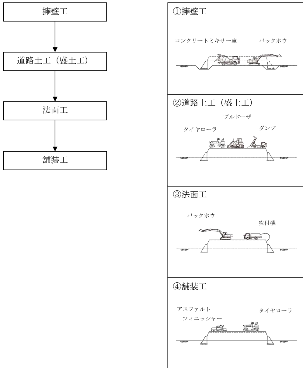
図 3.2.13-1 土工工事(盛土)の施工順序
