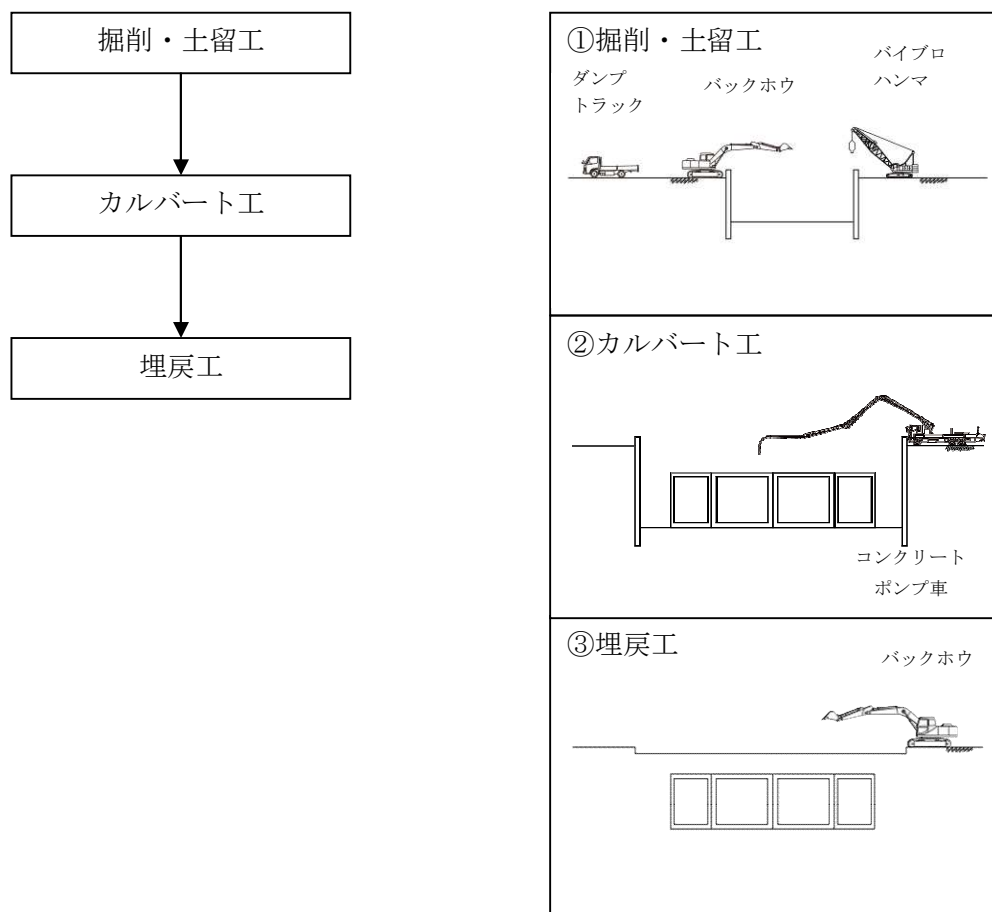
図 3.2.13-4 土工工事（トンネル部）の施工順序
