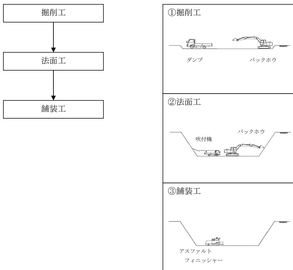
図 3.2.13-2 土工工事（切土部）の施工順序
