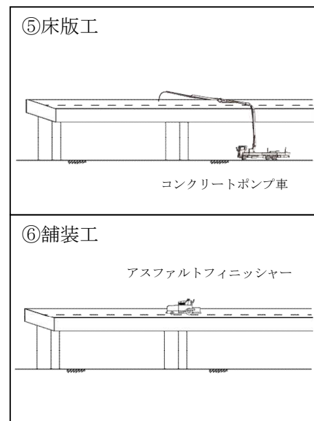
図 3.2.13-5(2)橋梁・高架工事の施工順序
