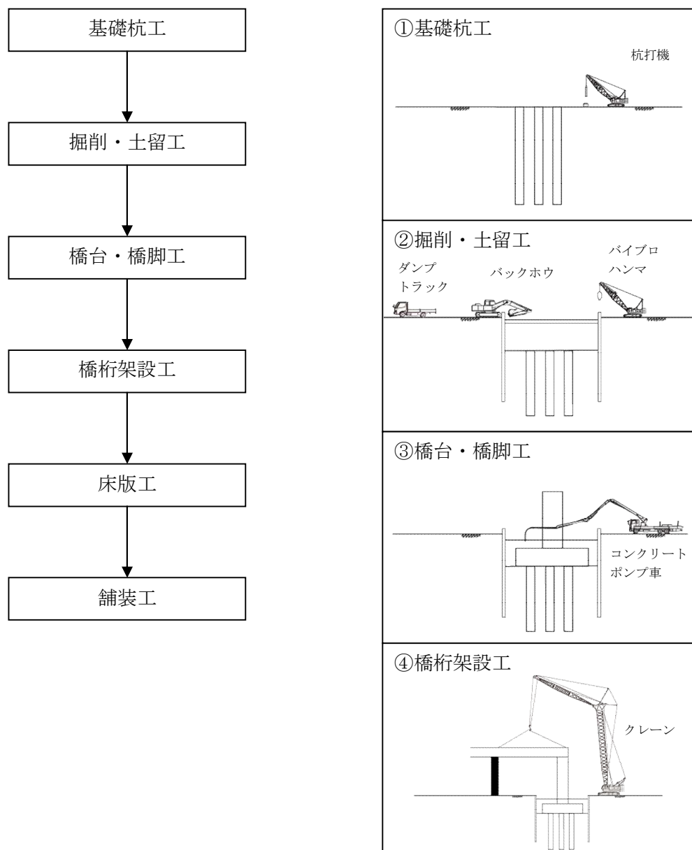
図 3.2.13-5(1)橋梁・高架工事の施工順序
