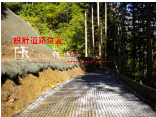
< 補強土壁工施工状況 >
