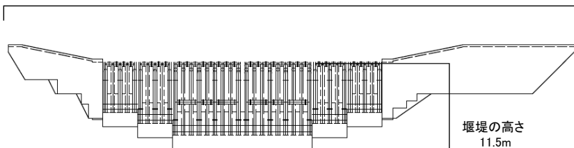
構造図 (正面より)
