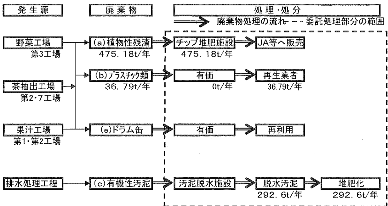
図5 廃棄物処理フロー図（現状）
