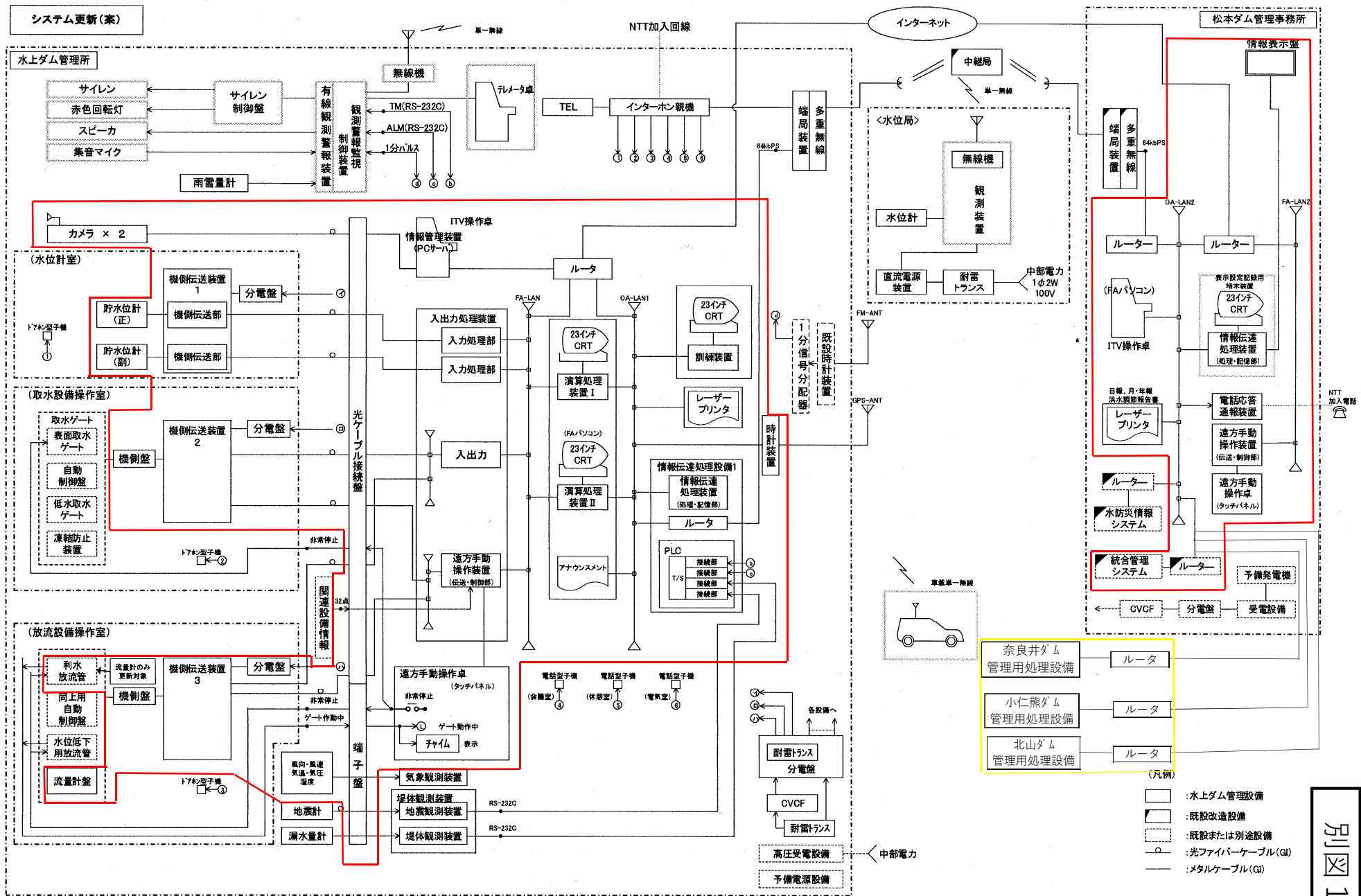
水上ダム管理設備システム構成図 (参考)
